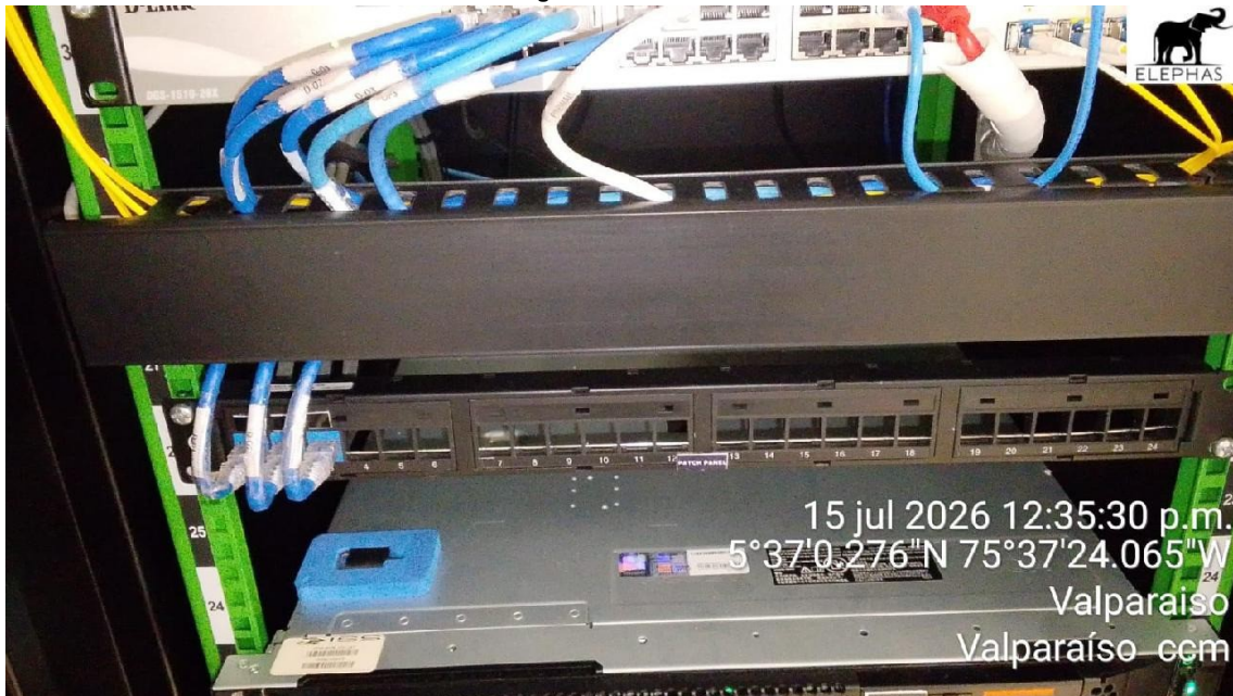
Foto organizador de cableado
