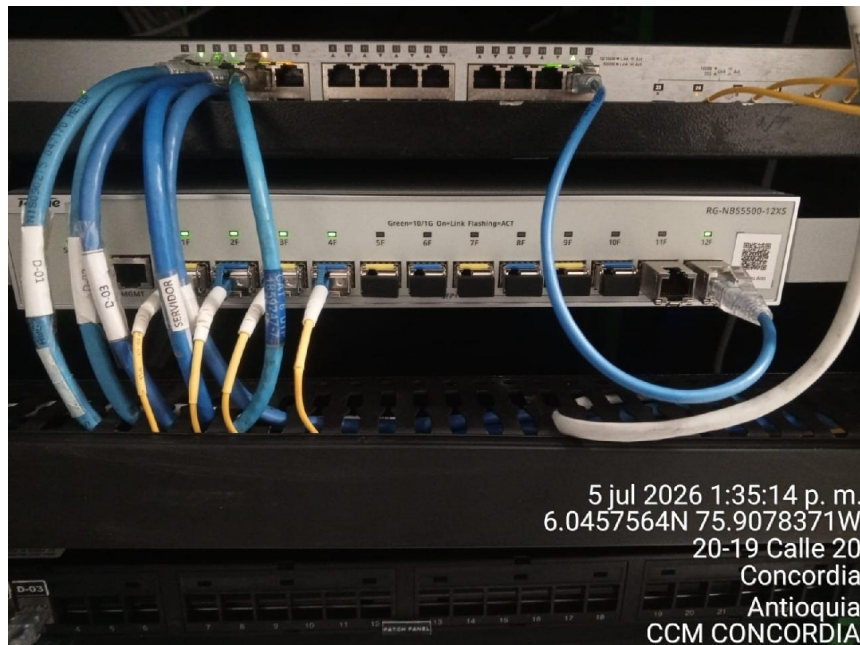
Foto switch
