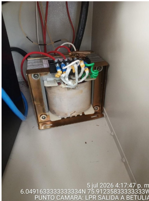
Foto Transformador Reductor
