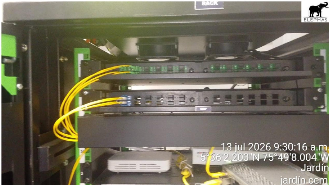
Foto ODF
