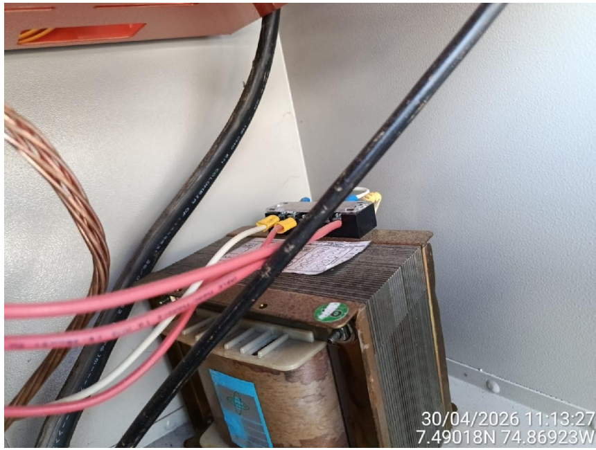
Foto Transformador Reductor
