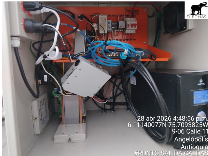
Foto Cables
