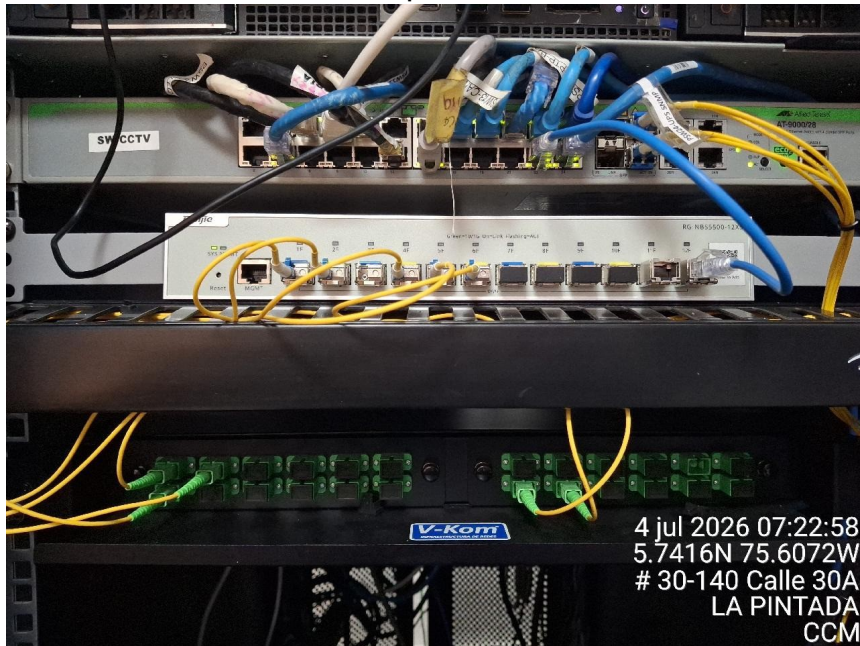
Foto patch cord
