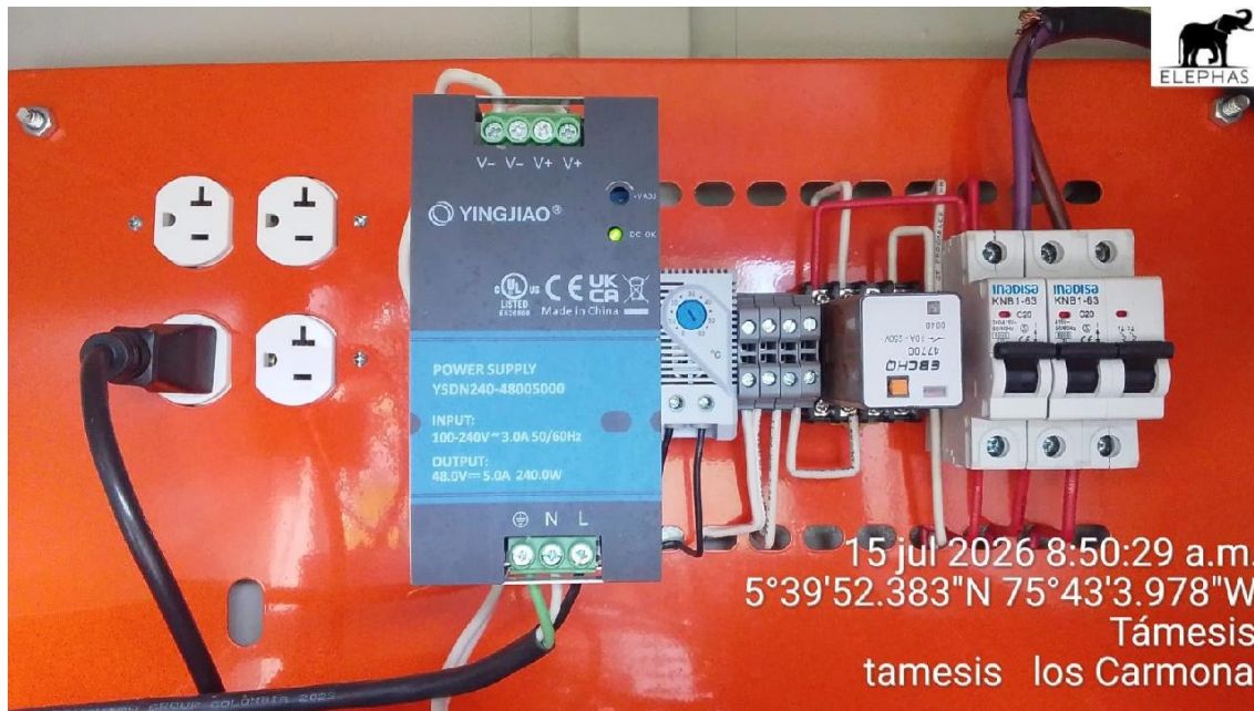
Foto Cables
