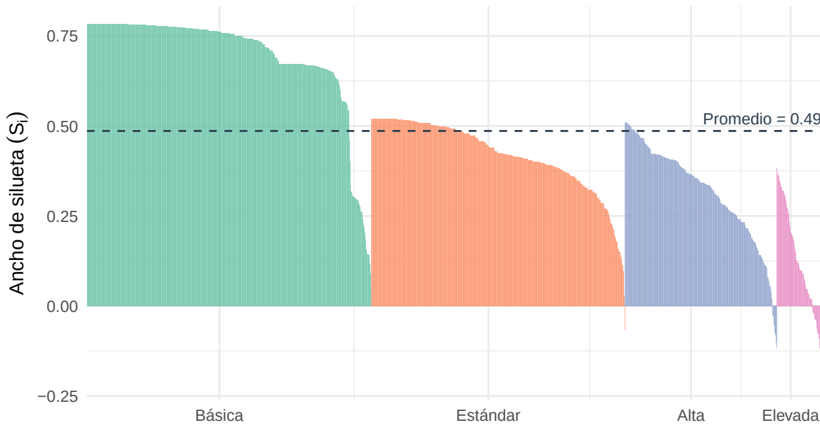
Figura 12: Gráfico de siluetas del agrupamiento k -means ( k = 4 ) sobre una submuestra de 1.500 propiedades de CABA. Cada barra es el ancho de silueta S_i de una propiedad, ordenadas dentro de cada segmento: valores cercanos a 1 indican una asignación nítida a su grupo, próximos a 0 una propiedad en la frontera entre segmentos, y negativos una posible mala asignación. La línea punteada marca el ancho de silueta promedio, medida global de la calidad del agrupamiento.
