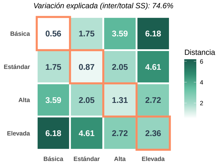
Figura 13: Matriz de distancias en el espacio estandarizado (superficie cubierta, ambientes, dormitorios y baños). La diagonal (recuadrada) mide la cohesión intra-clúster como distancia media de las propiedades a su centroide; fuera de la diagonal, la separación inter-clúster entre centroides. Valores bajos en la diagonal y altos fuera de ella indican grupos compactos y bien separados.
