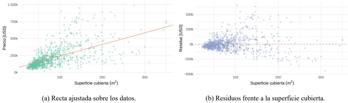
Figura 7: Regresión lineal simple del precio sobre la superficie cubierta (muestra aleatoria de 15.000 propiedades).
