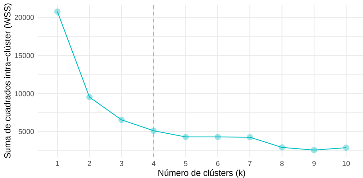
Figura 10: Método del codo: suma de cuadrados intra-clúster (WSS) en función del número de clústeres k.
