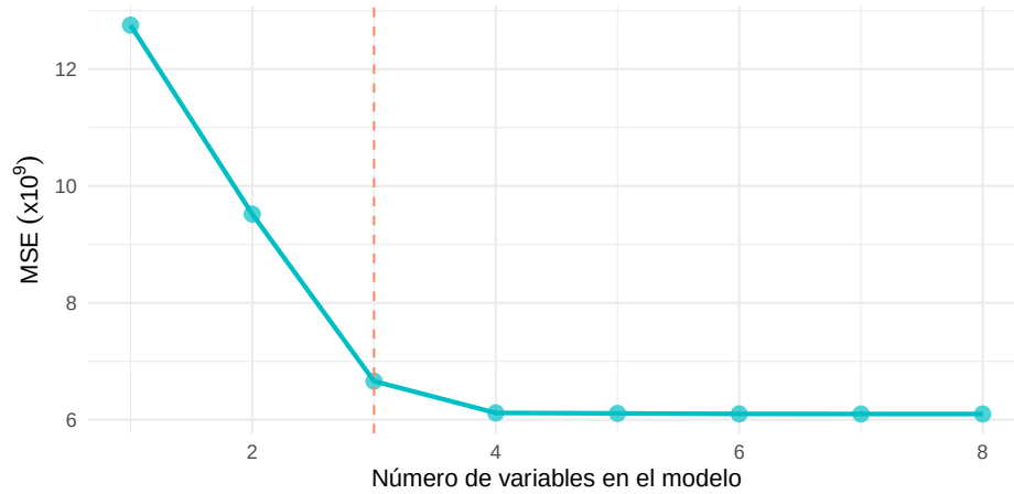
Figura 8: Error cuadrático medio de validación cruzada según el número de variables incluidas en el modelo de RLM.
