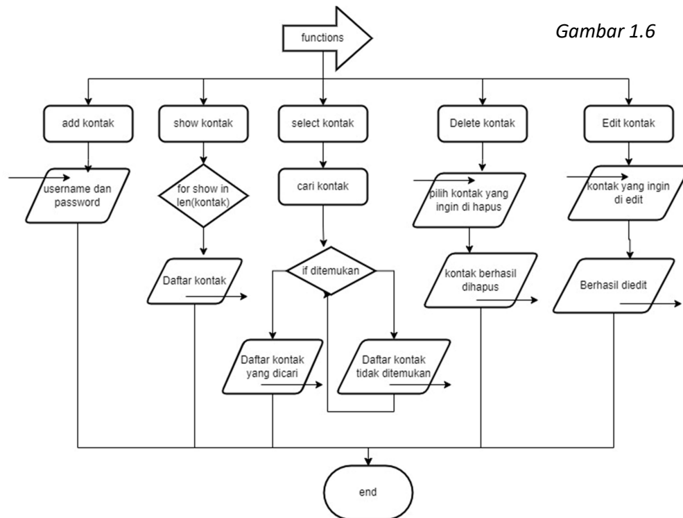
Gambar (flowcart menu tambah, lihat, cari, hapus, dan edit kontak yang fungsinya dipanggil pada program admin, user, dan tamu pada menu login)
