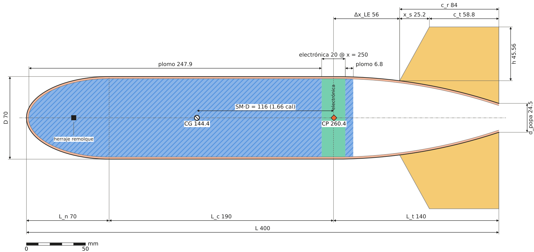
VISTA LATERAL EN CORTE (aletas en verdadera magnitud)
