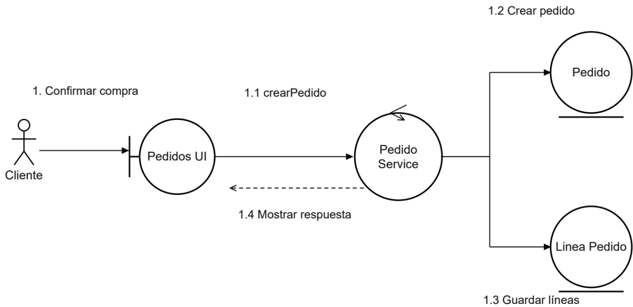
Flujo principal de CU14.
