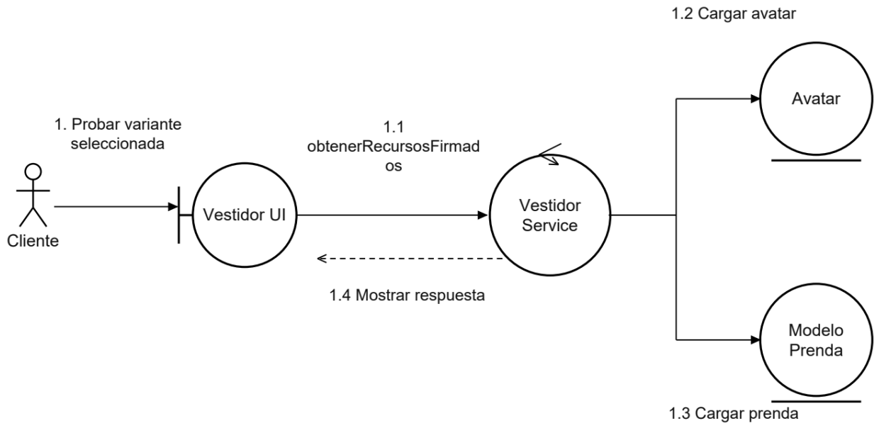
Flujo principal de CU16.
