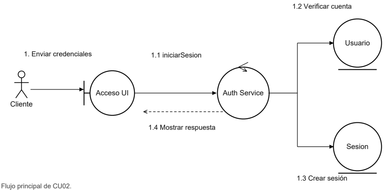
Flujo principal de CU02. Figura 41. CU02 Diagrama de comunicación
