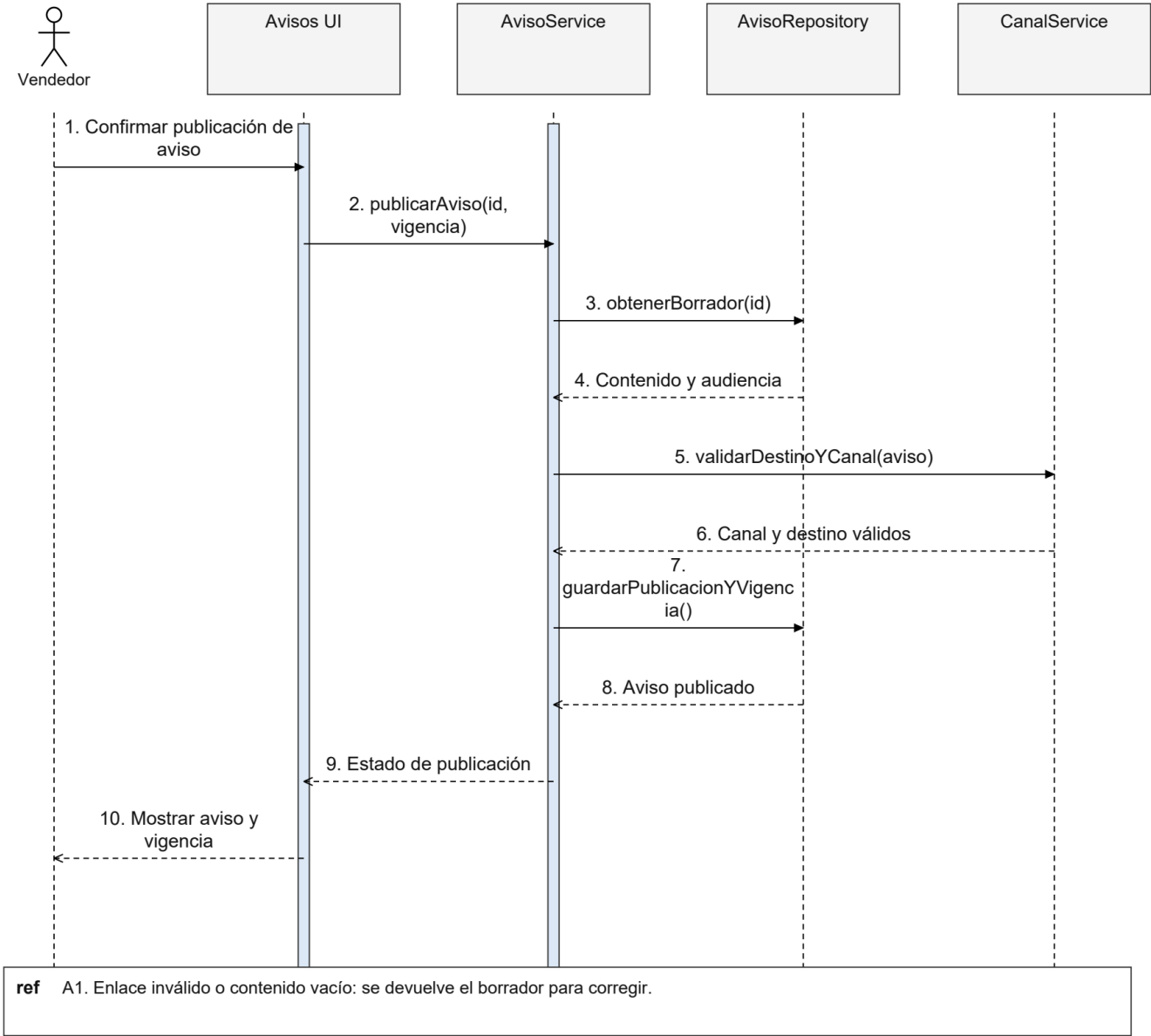
Figura 105. CU06 Secuencia de diseño
