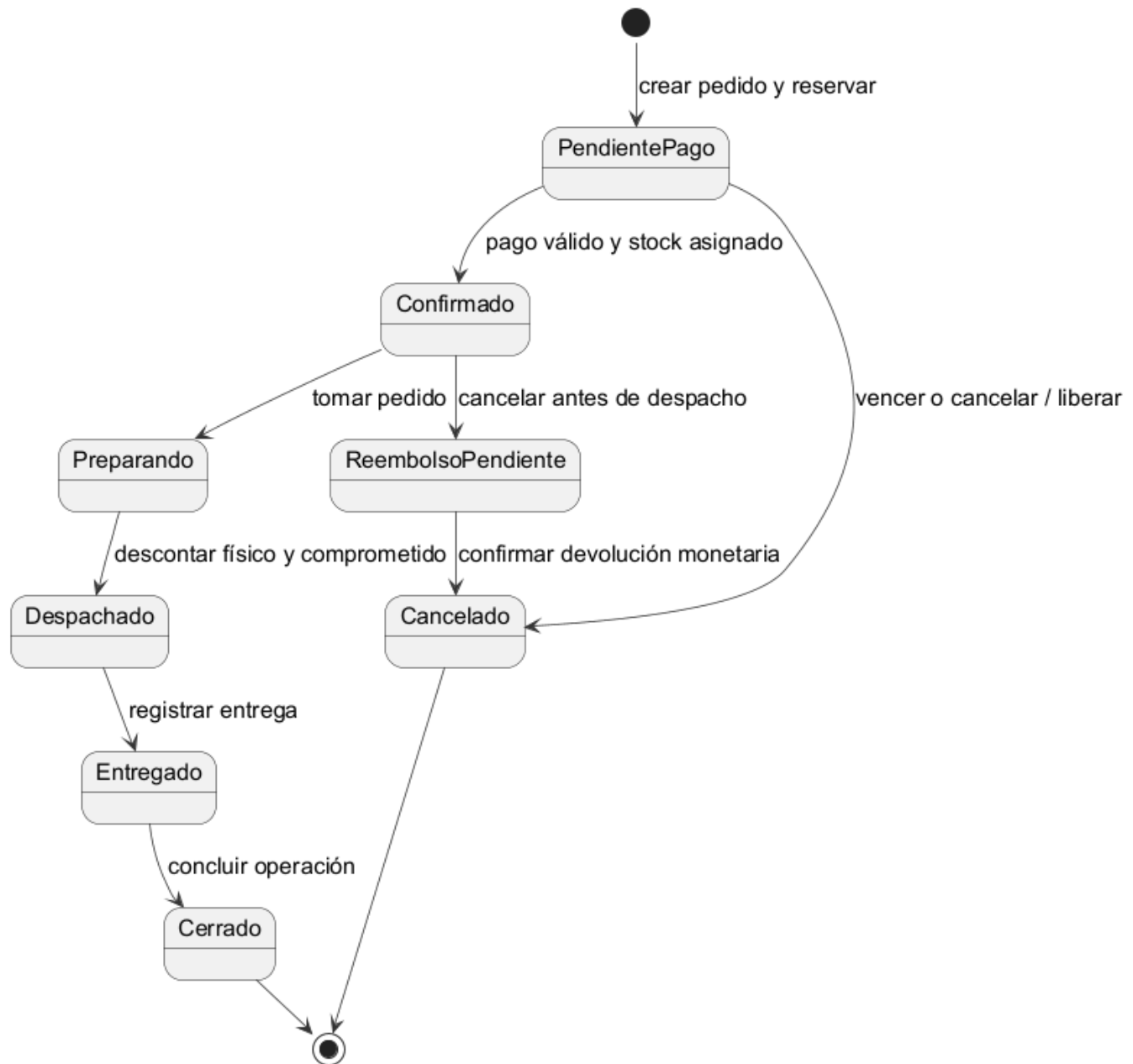
Figura 93. Estados comerciales y principales transiciones del pedido
