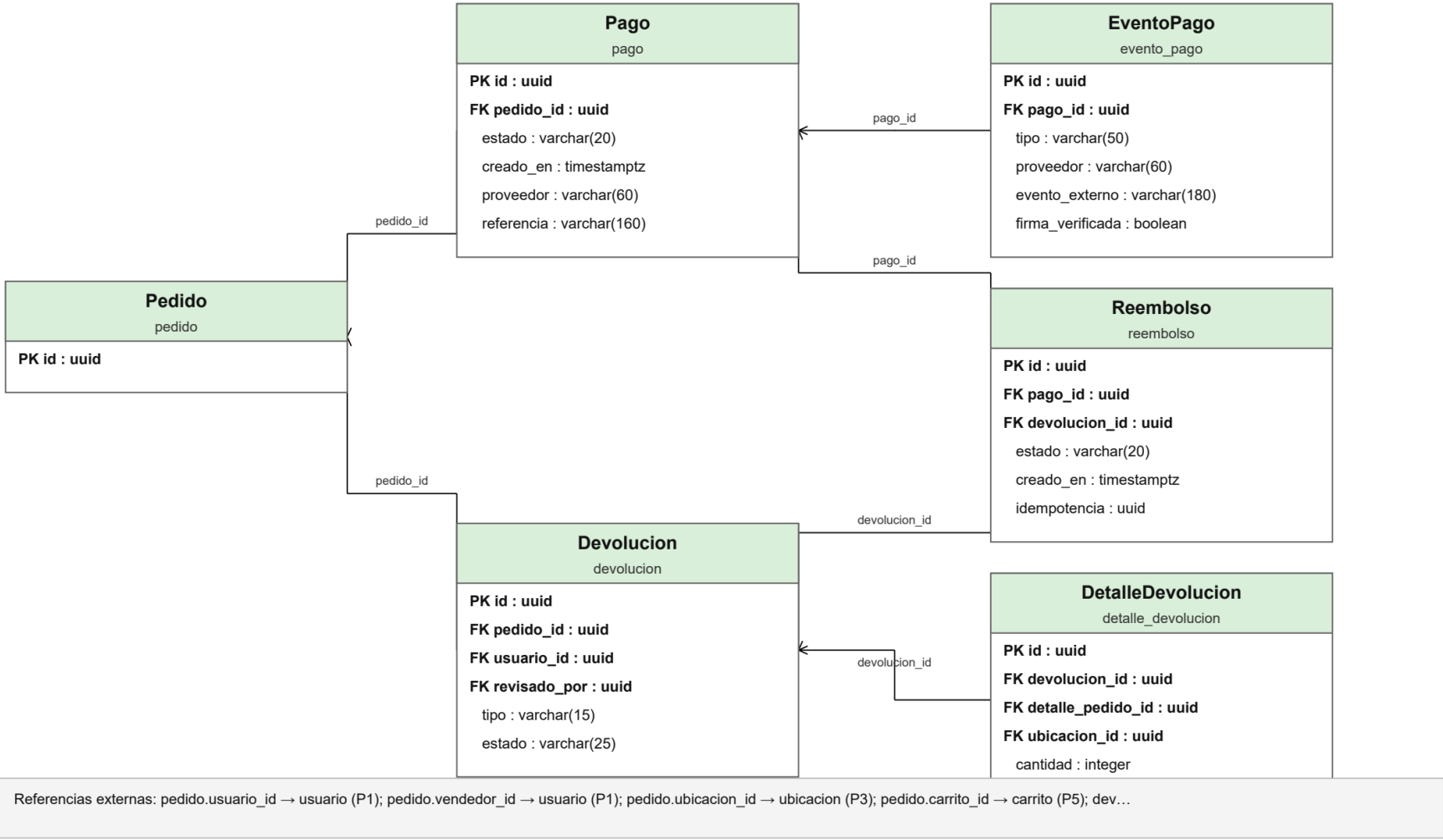
Figura 125. P5 Pagos devoluciones y reembolsos
