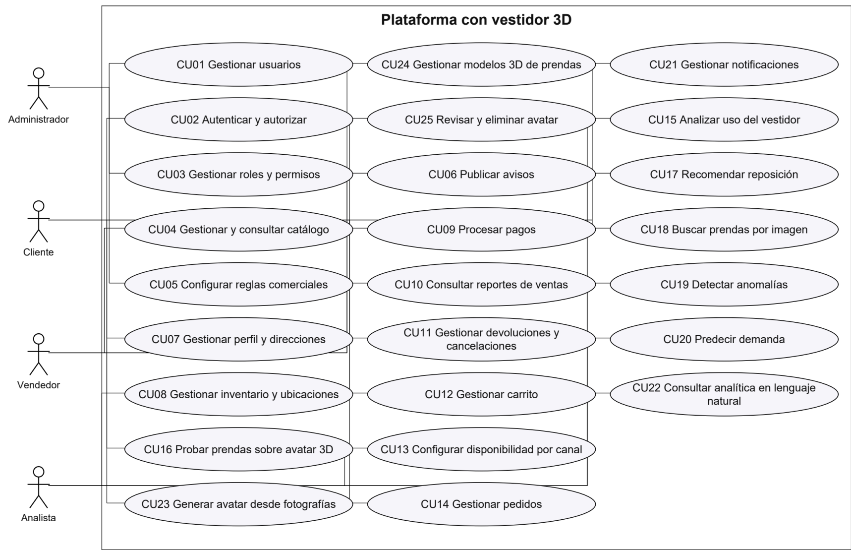
Figura 30. Vista general con el actor principal de cada caso
