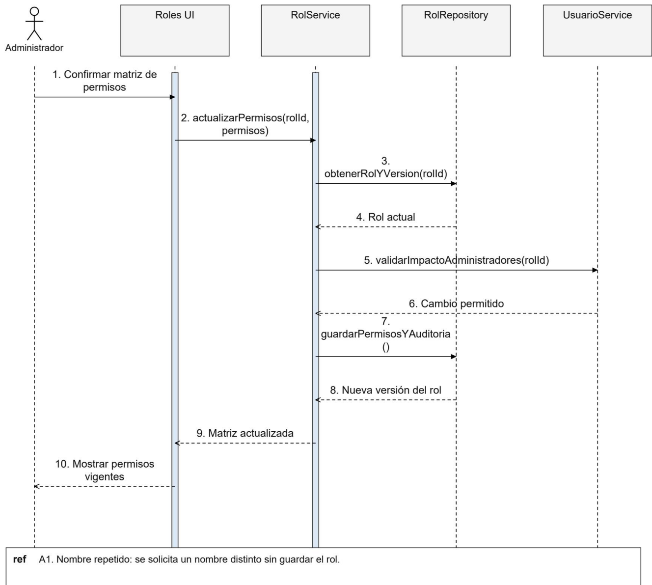
Figura 96. CU03 Secuencia de diseño
