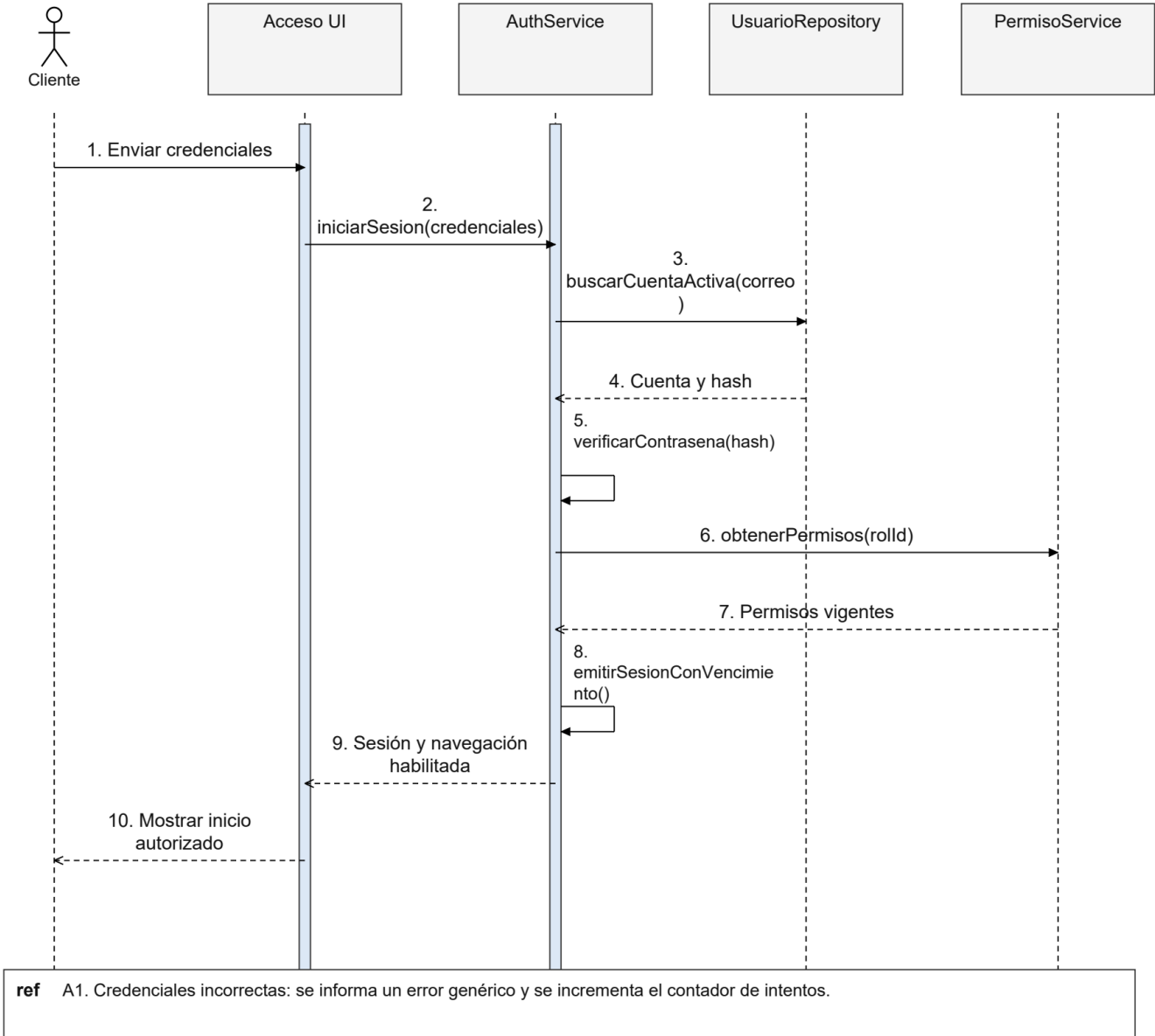
Figura 95. CU02 Secuencia de diseño
