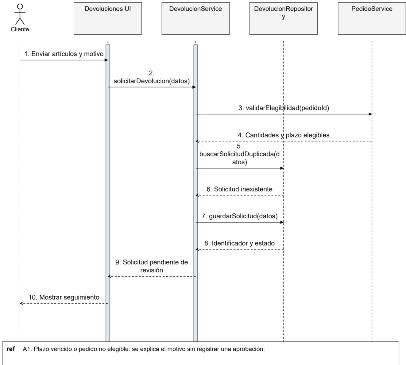
Figura 108. CU11 Secuencia de diseño
