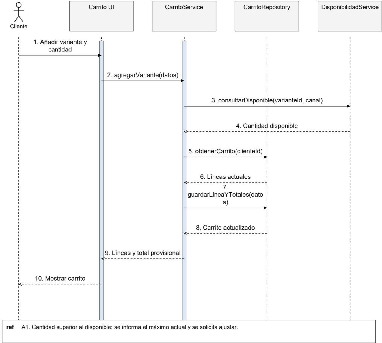
Figura 109. CU12 Secuencia de diseño
