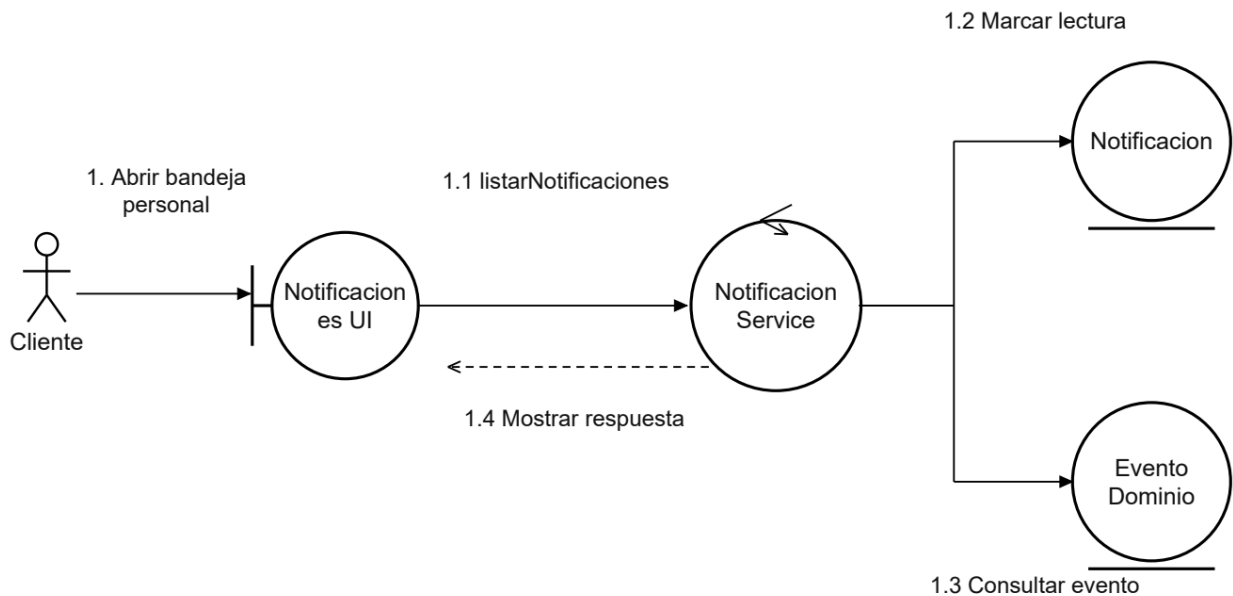
Figura 75. CU21 Diagrama de comunicación
