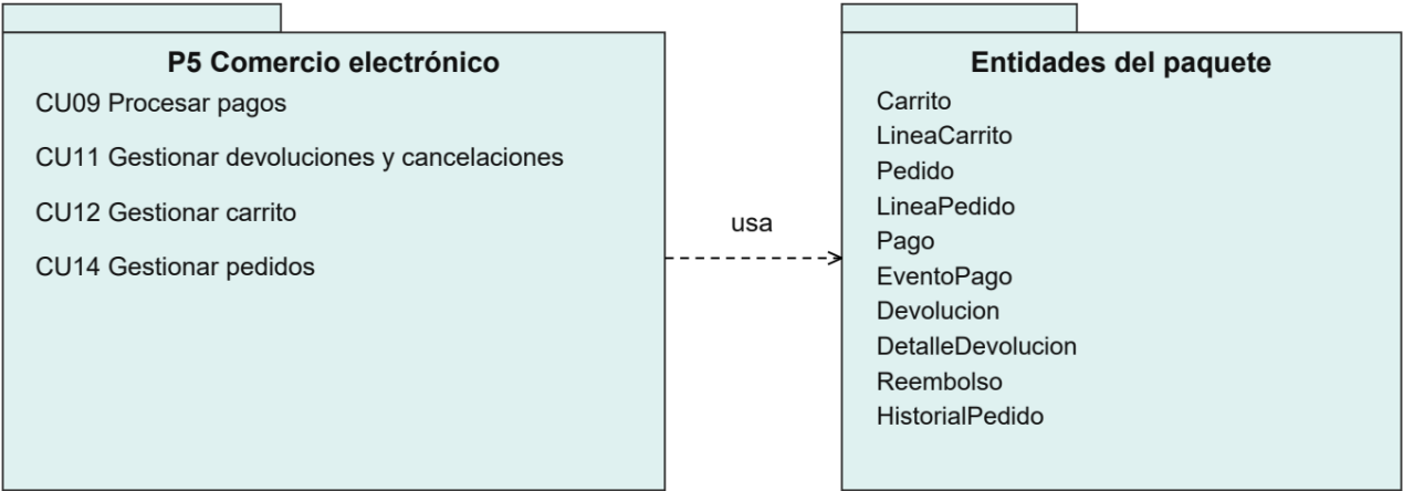
Figura 35. Vista del paquete P5
