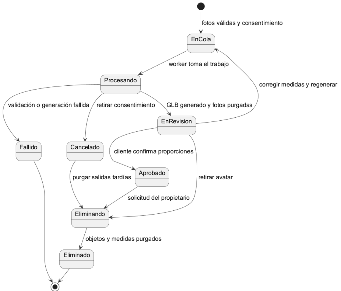
Figura 92. Ciclo de vida del trabajo y la versión de avatar
