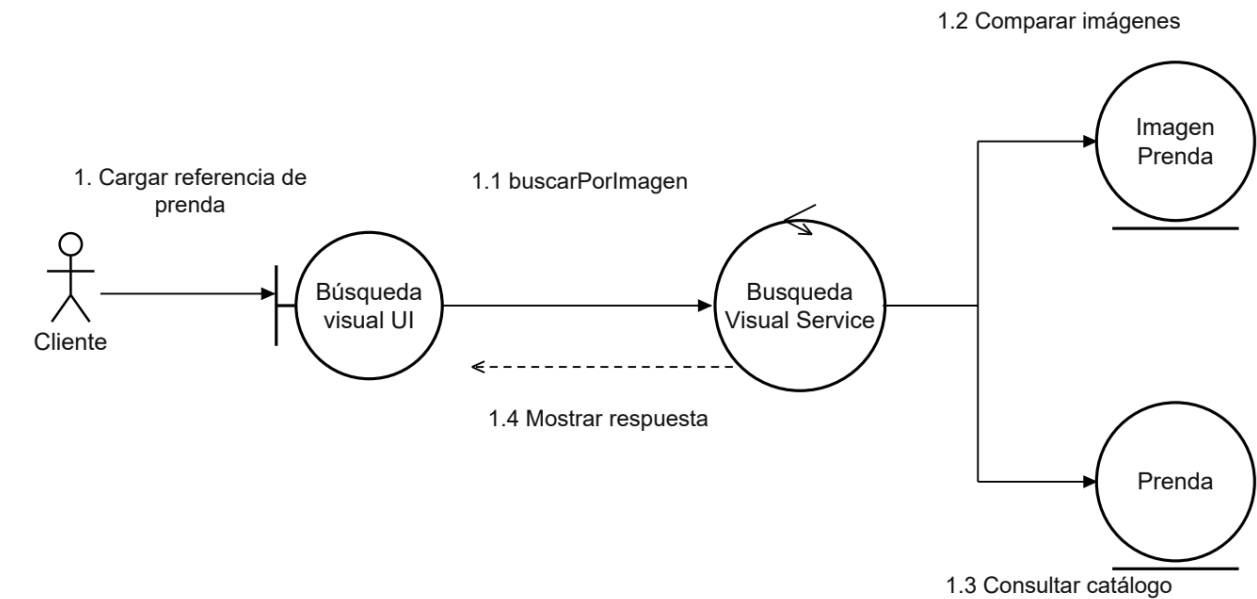
Figura 81. CU18 Diagrama de comunicación
