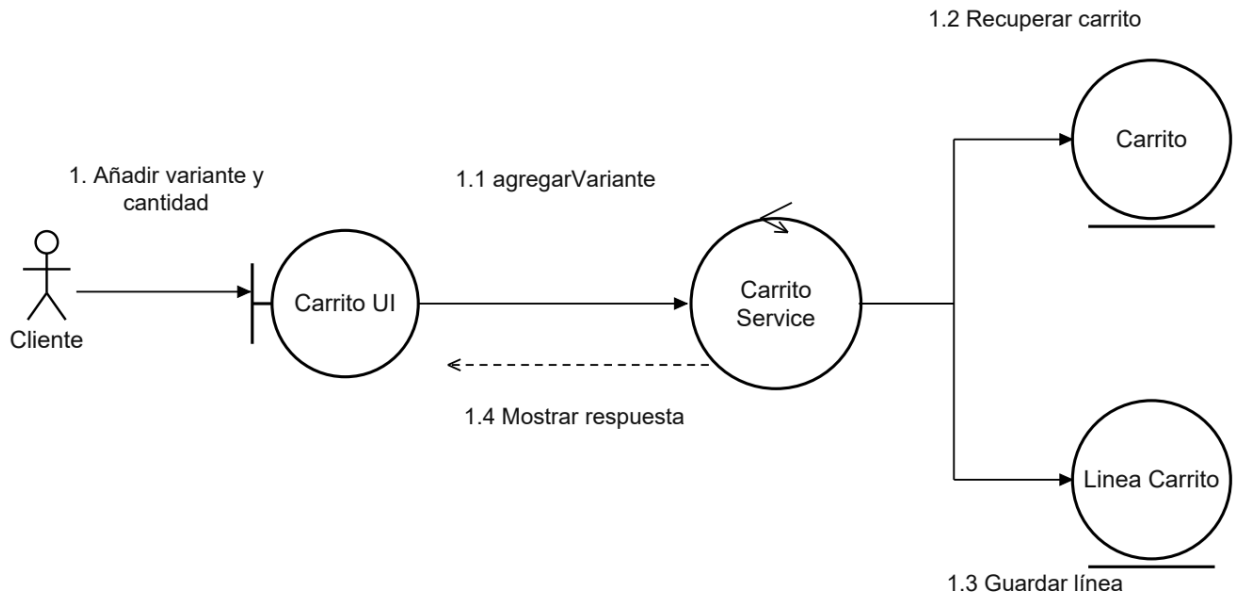
Figura 69. CU12 Diagrama de comunicación
