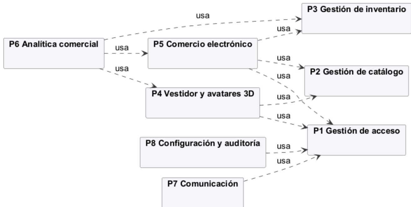
Figura 89. Dependencias dirigidas hacia los paquetes proveedores
