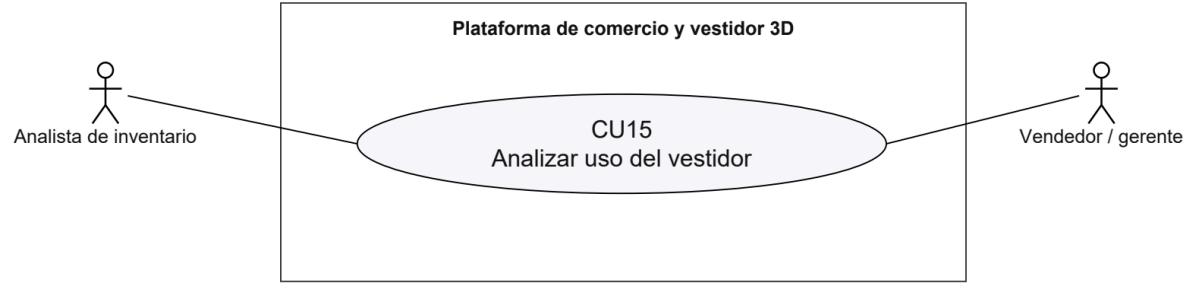
Figura 21. CU15 Actores y caso de uso
