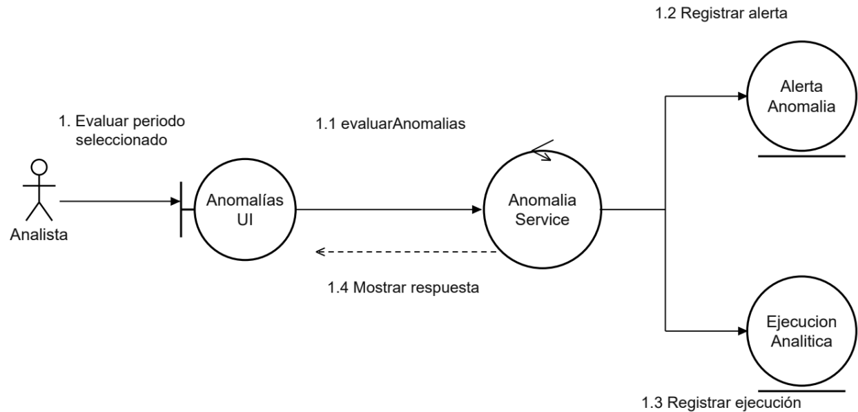
Figura 83. CU19 Diagrama de comunicación
