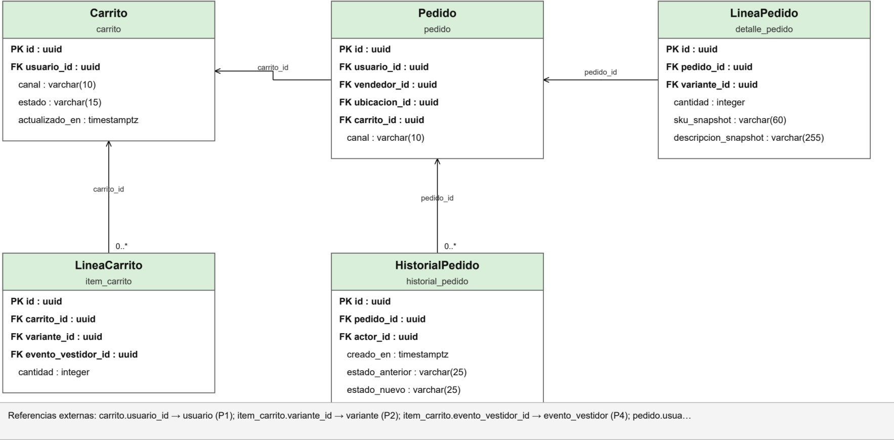
Figura 124. P5 Carrito pedidos e historial
