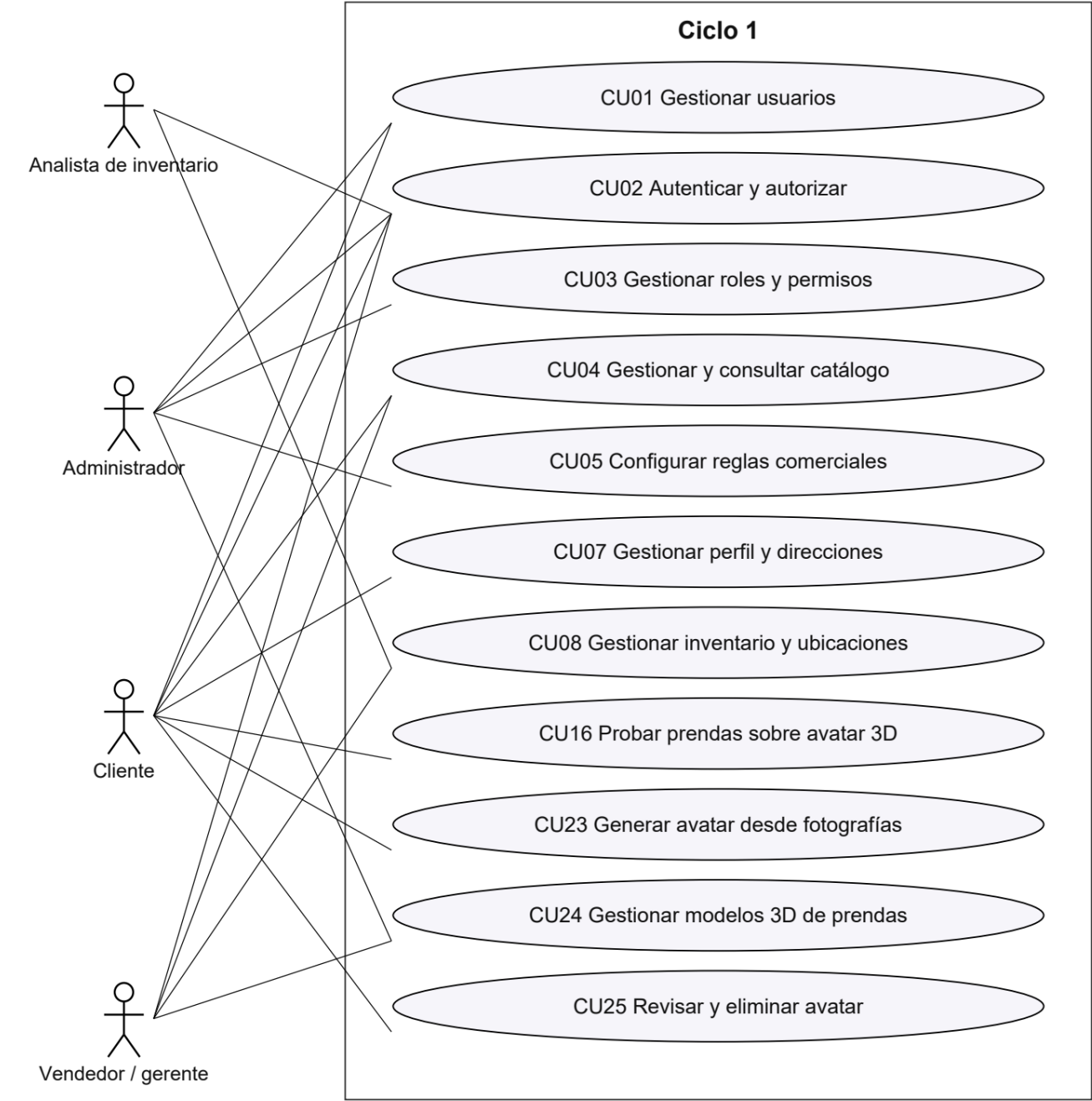
Figura 27. Asociaciones de actores y casos del ciclo 1
