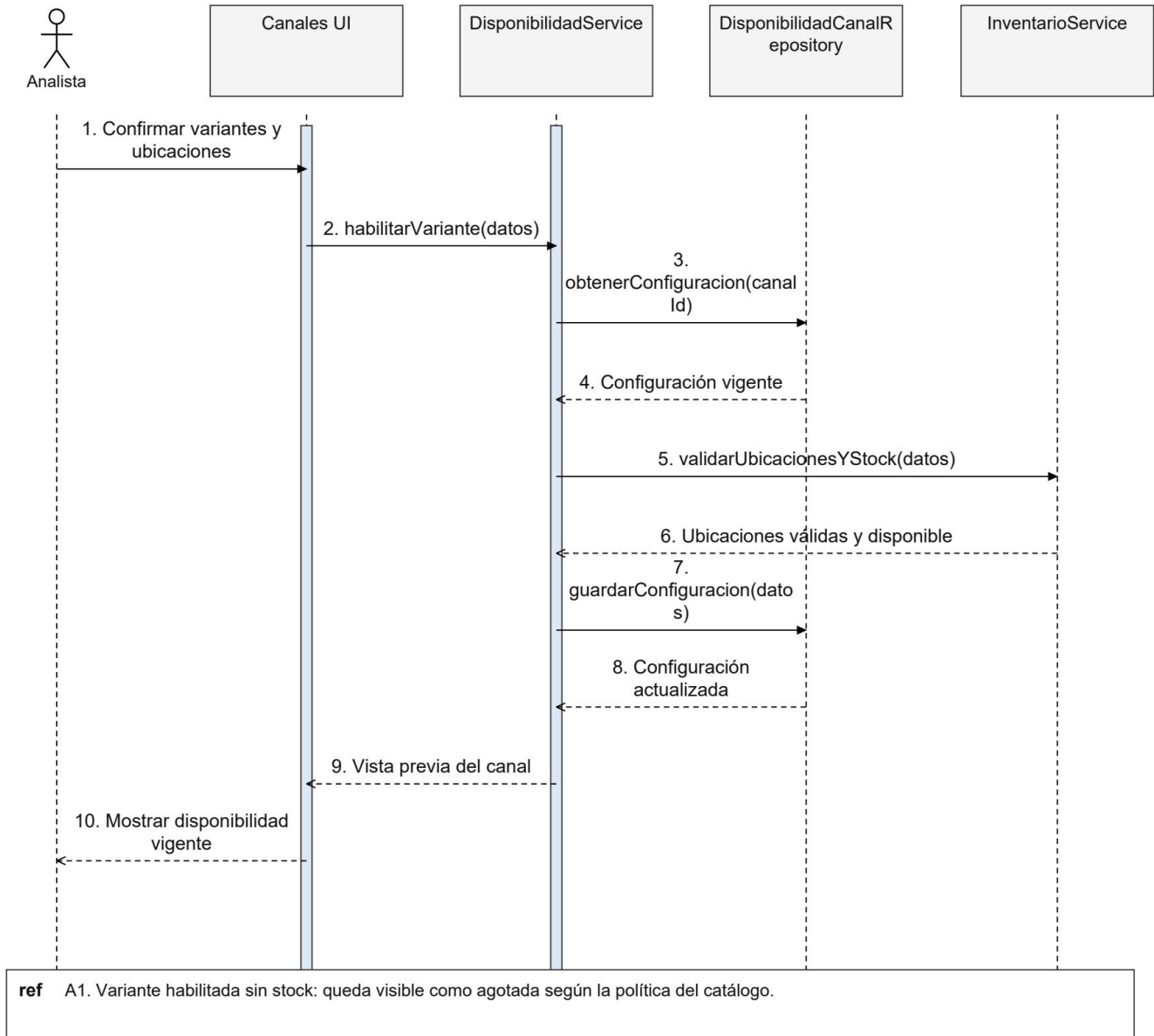
Figura 110. CU13 Secuencia de diseño
