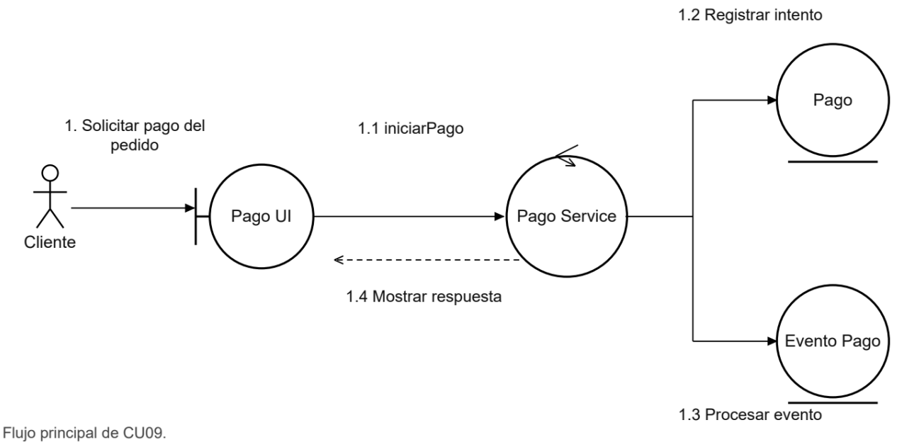
Figura 63. CU09 Diagrama de comunicación
