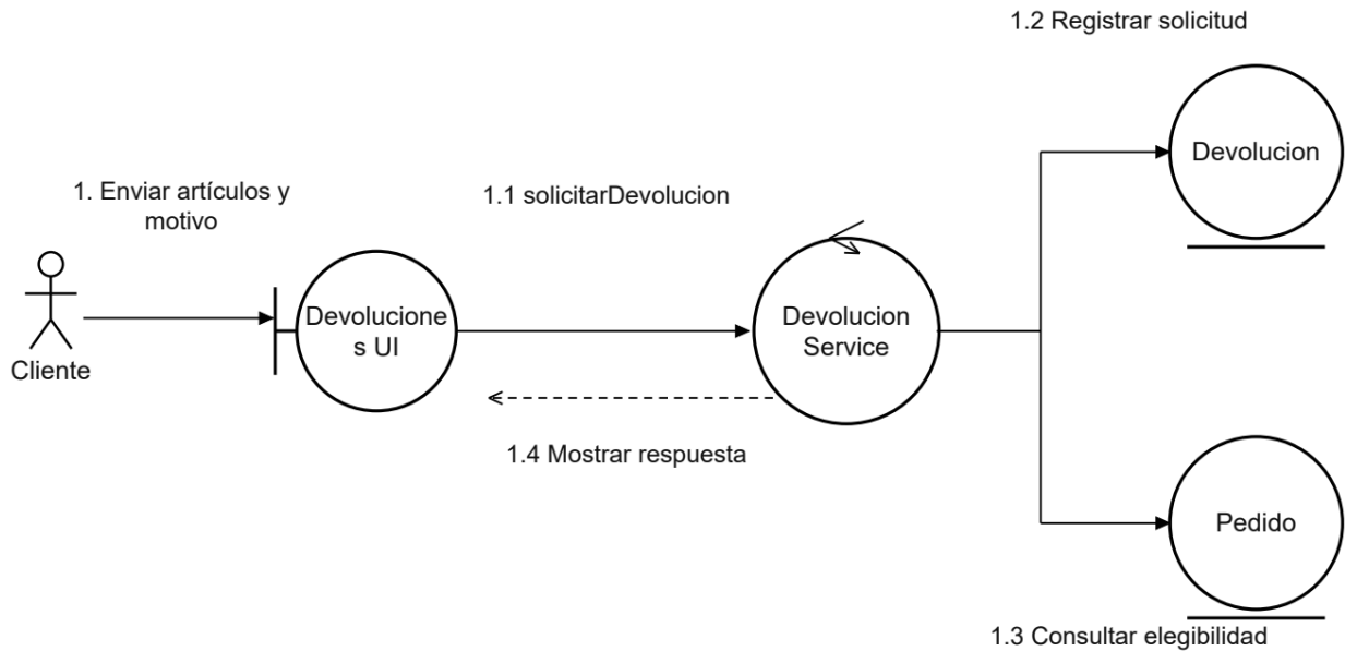
Figura 67. CU11 Diagrama de comunicación
