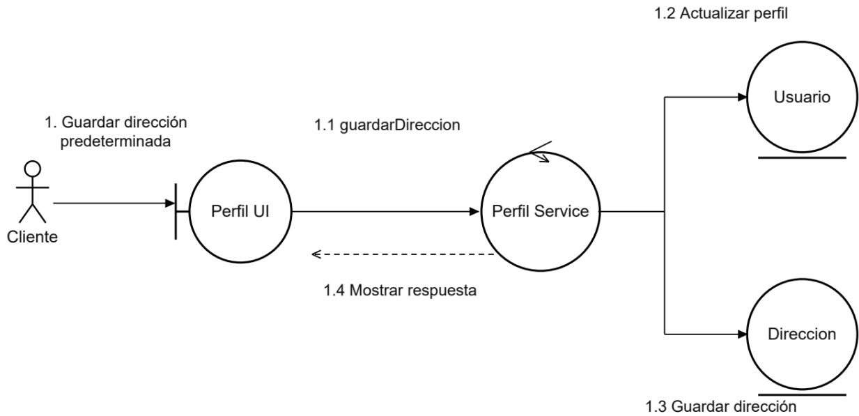
Figura 49. CU07 Diagrama de comunicación
