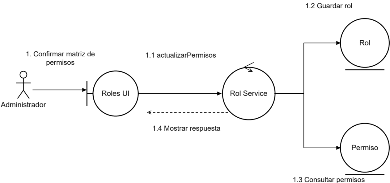
Figura 43. CU03 Diagrama de comunicación
