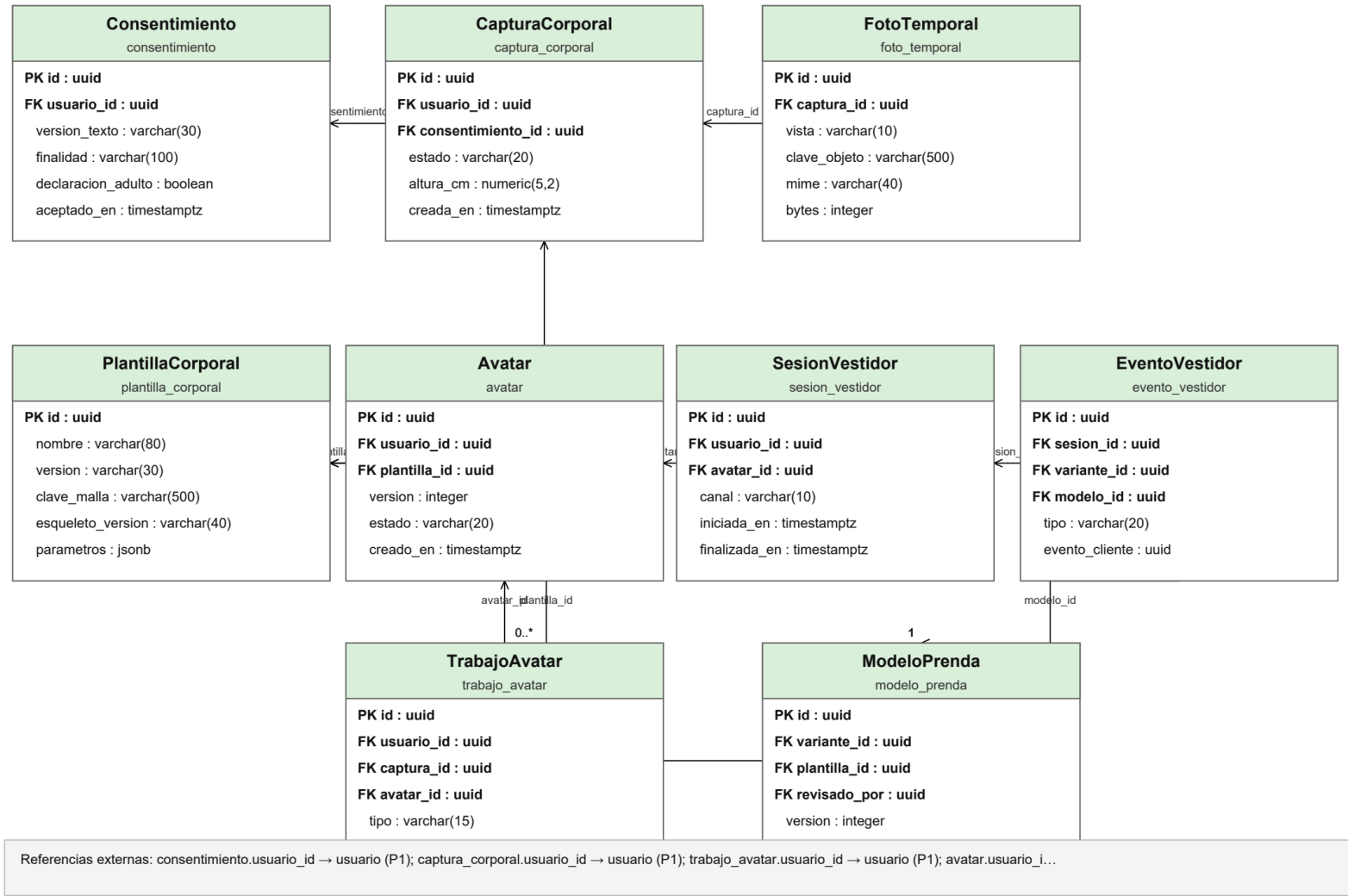
Figura 123. P4 Modelo lógico ordenado
