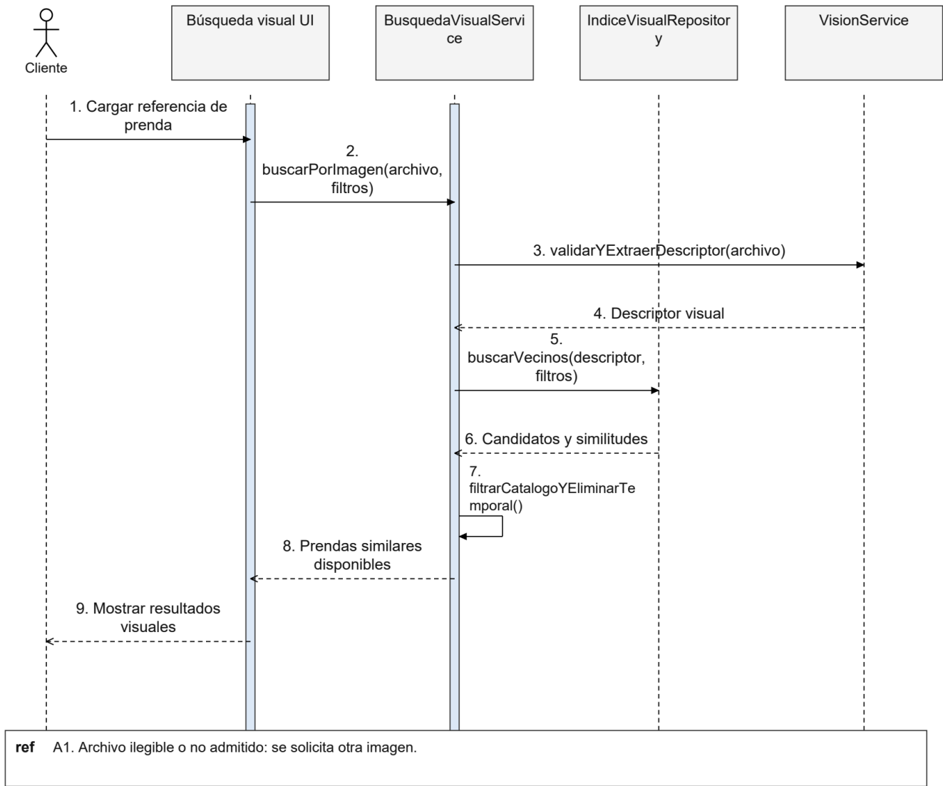
Figura 115. CU18 Secuencia de diseño
