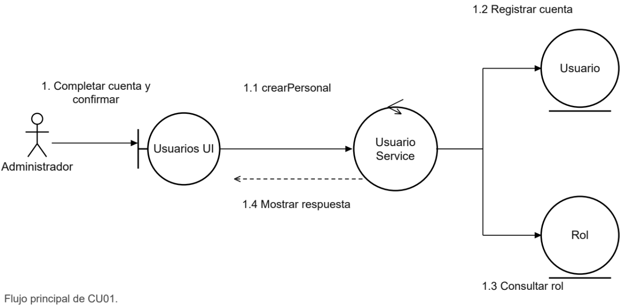
Figura 39. CU01 Diagrama de comunicación
