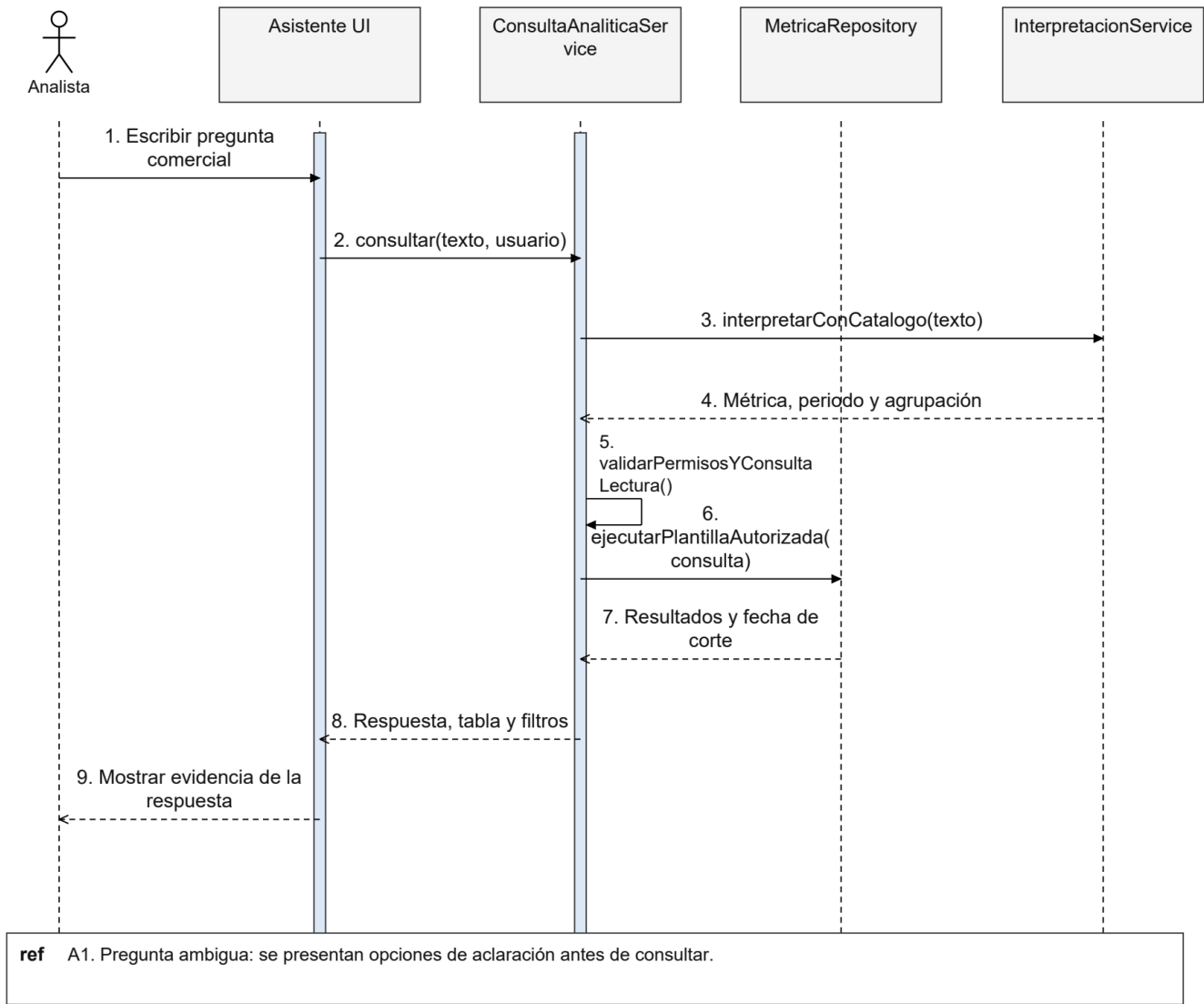
Figura 118. CU22 Secuencia de diseño
