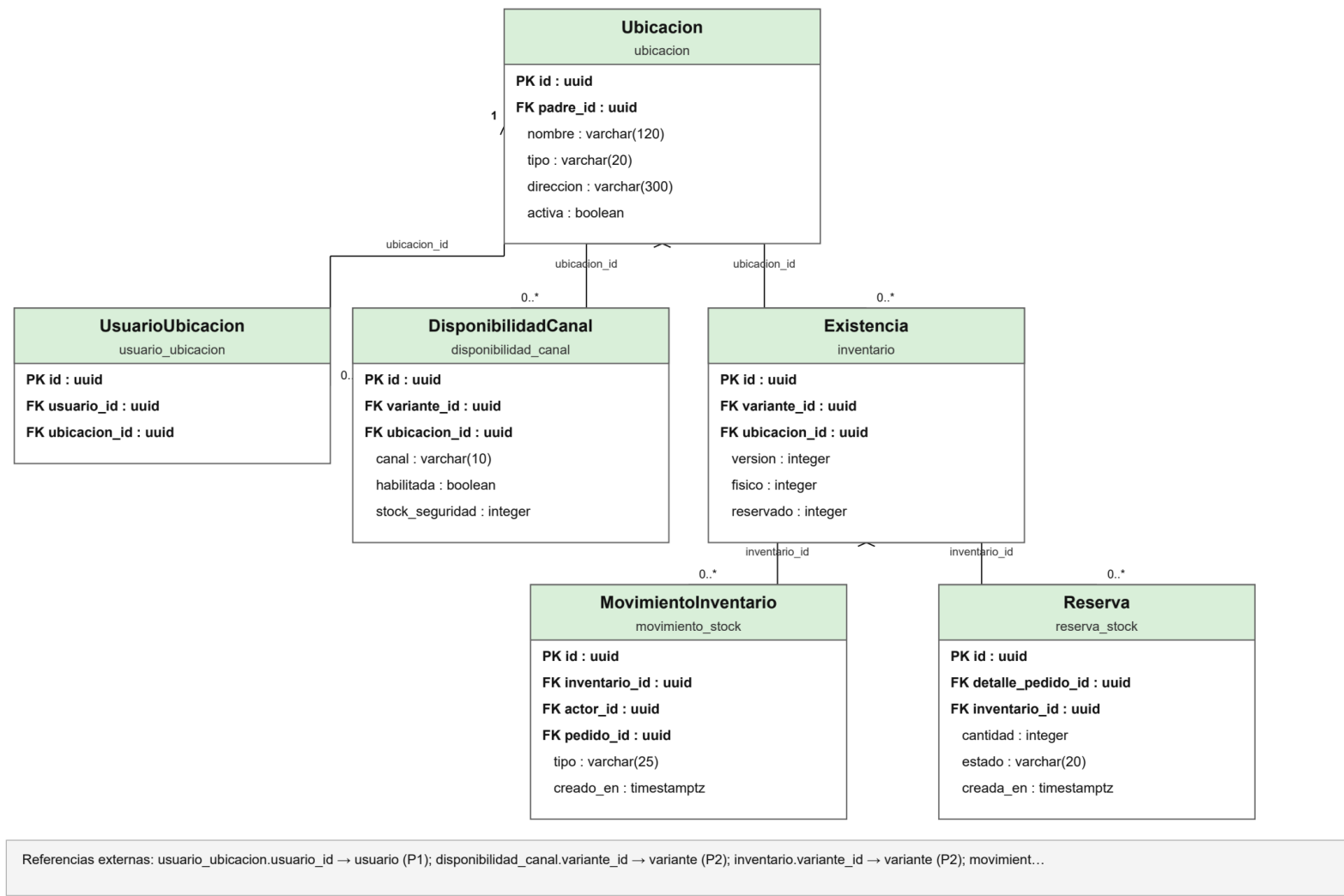
Figura 122. P3 Modelo lógico ordenado
