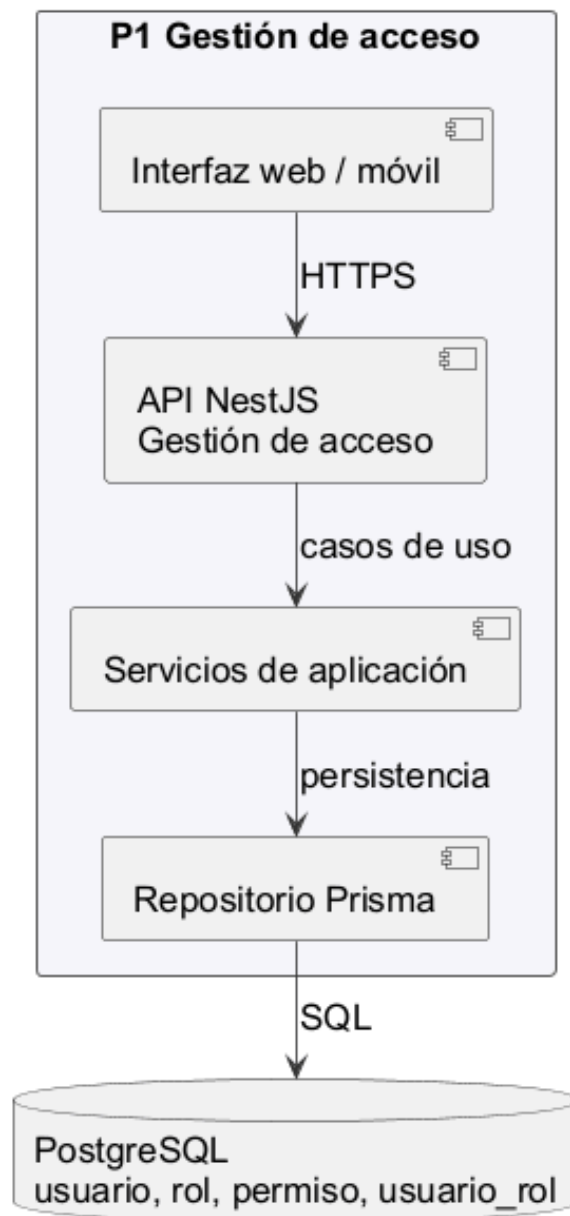
Figura 129. Componentes previstos del paquete P1
