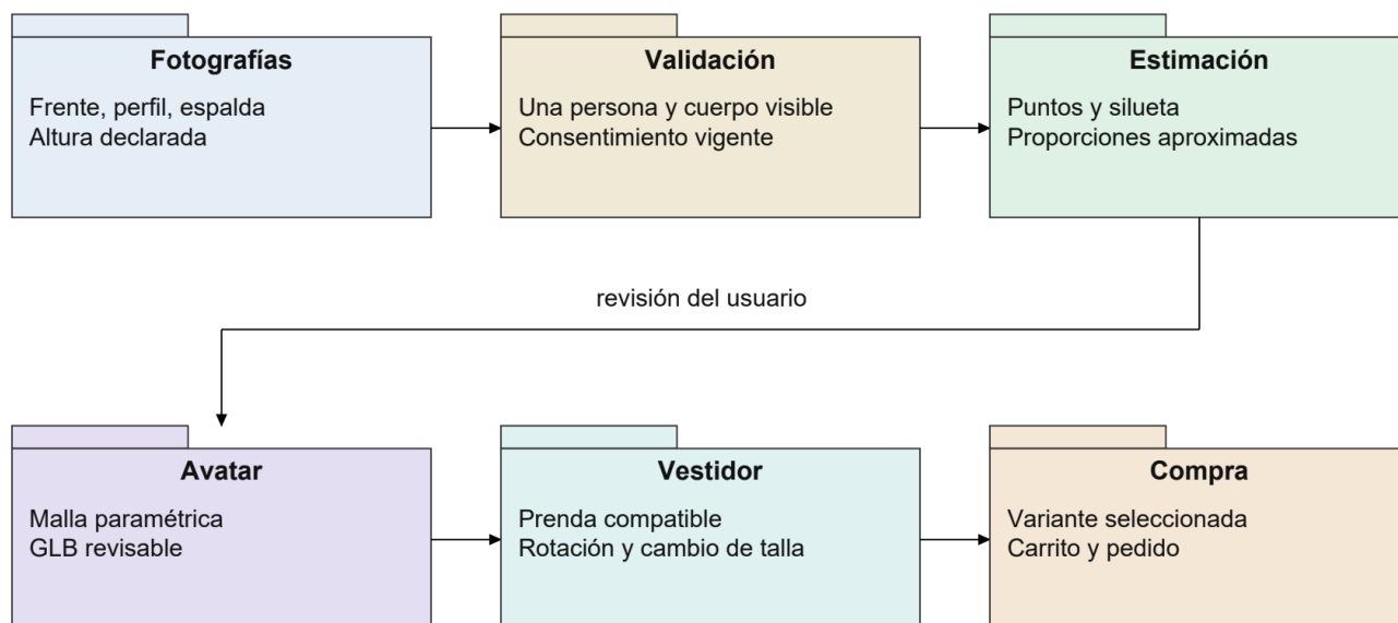
Figura 1. Flujo de fotografías, avatar, vestidor y compra
