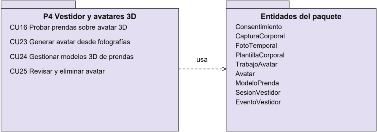
Figura 34. Vista del paquete P4
