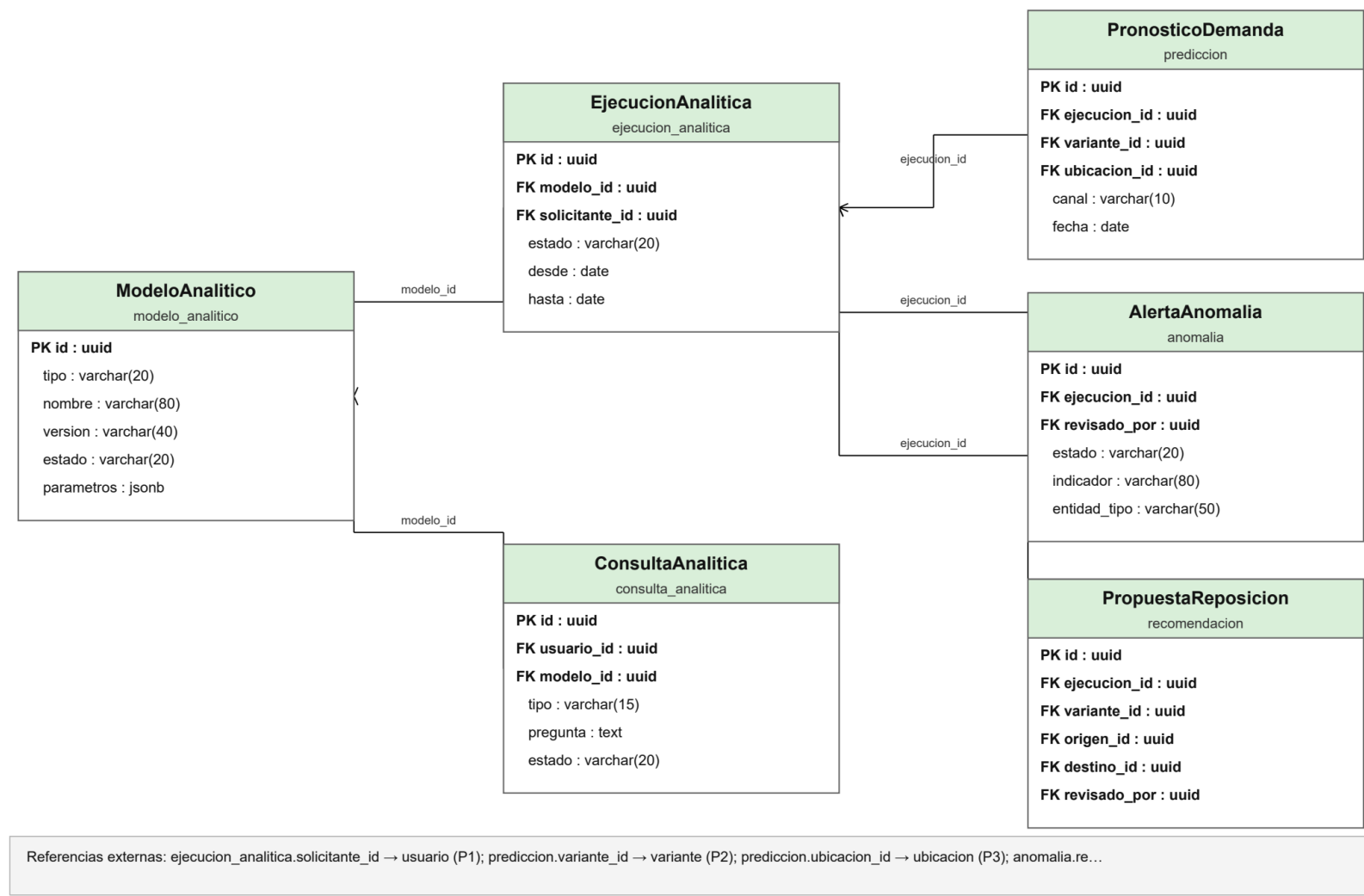
Figura 126. P6 Modelo lógico ordenado
