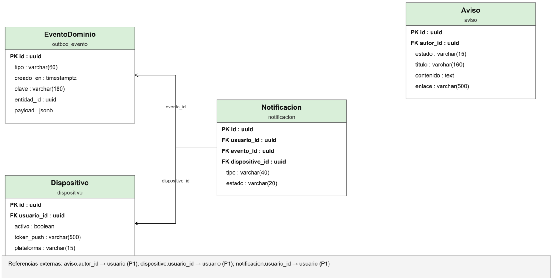
Figura 127. P7 Modelo lógico ordenado
