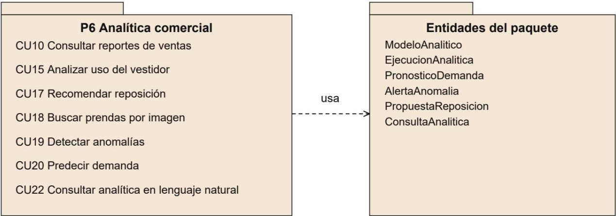
Figura 36. Vista del paquete P6
