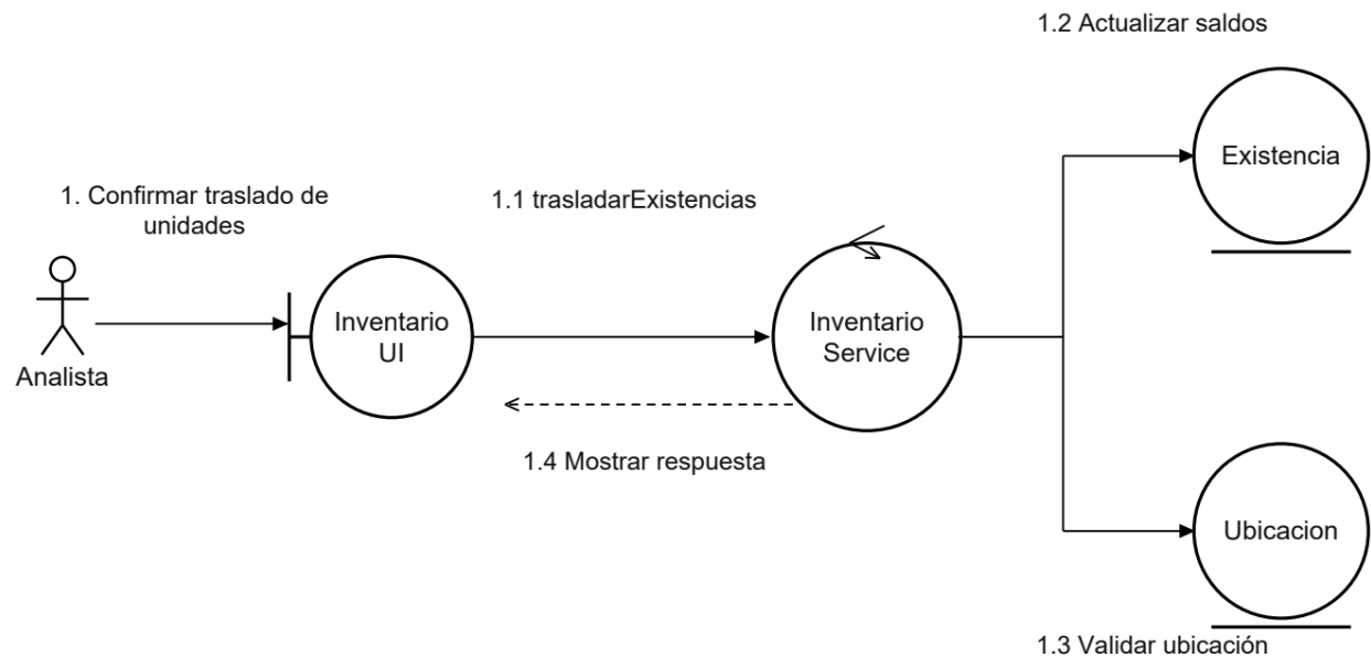
Figura 51. CU08 Diagrama de comunicación
