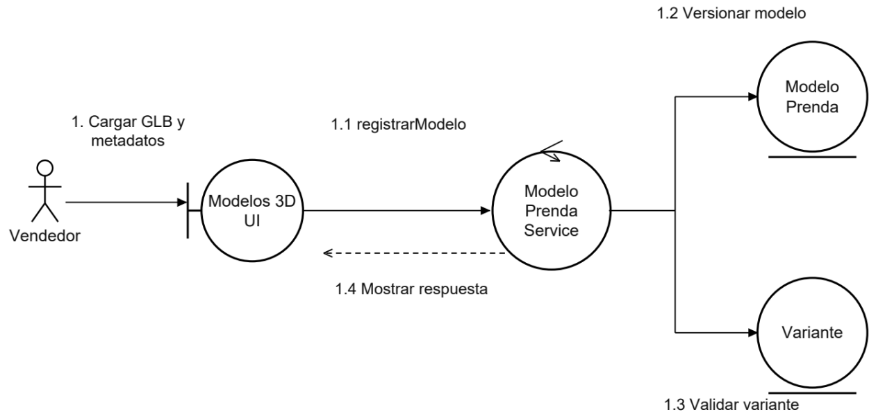
Figura 57. CU24 Diagrama de comunicación
