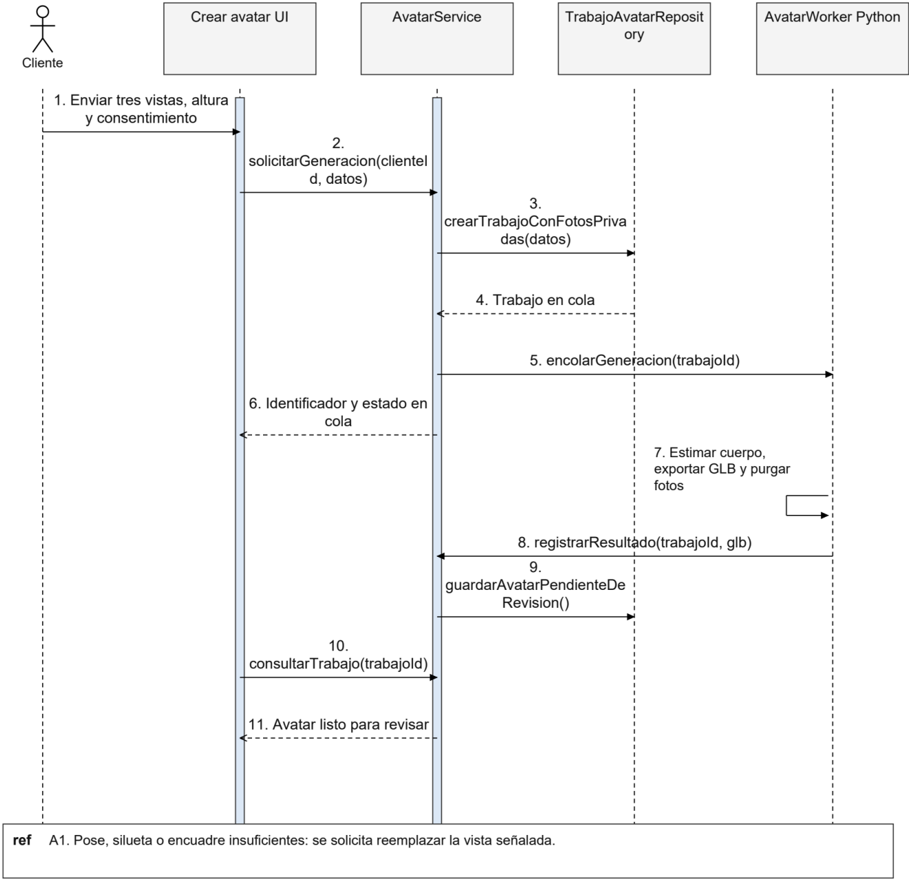
Figura 102. CU23 Secuencia de diseño
