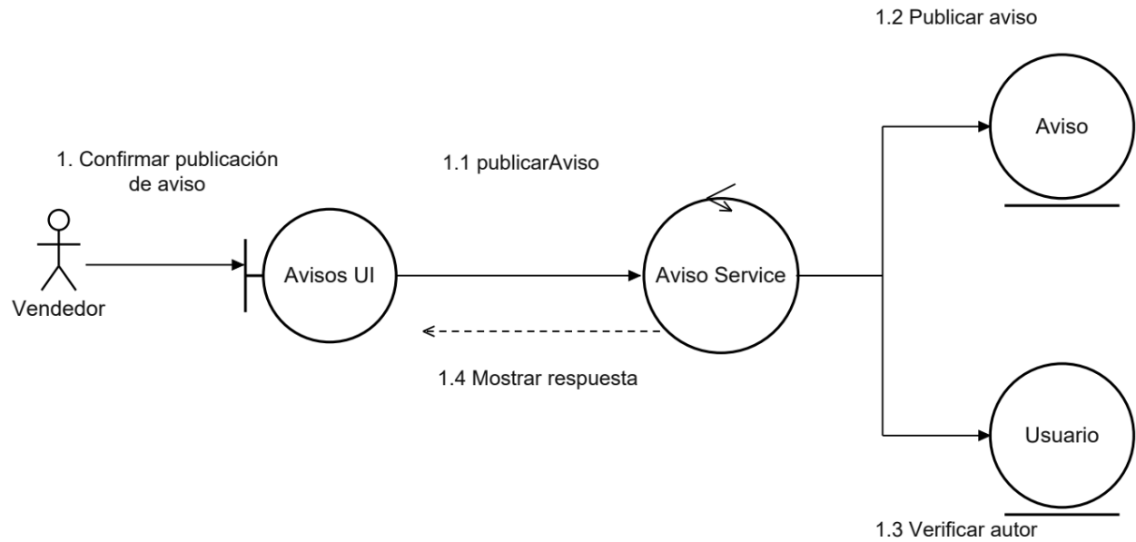
Figura 61. CU06 Diagrama de comunicación
