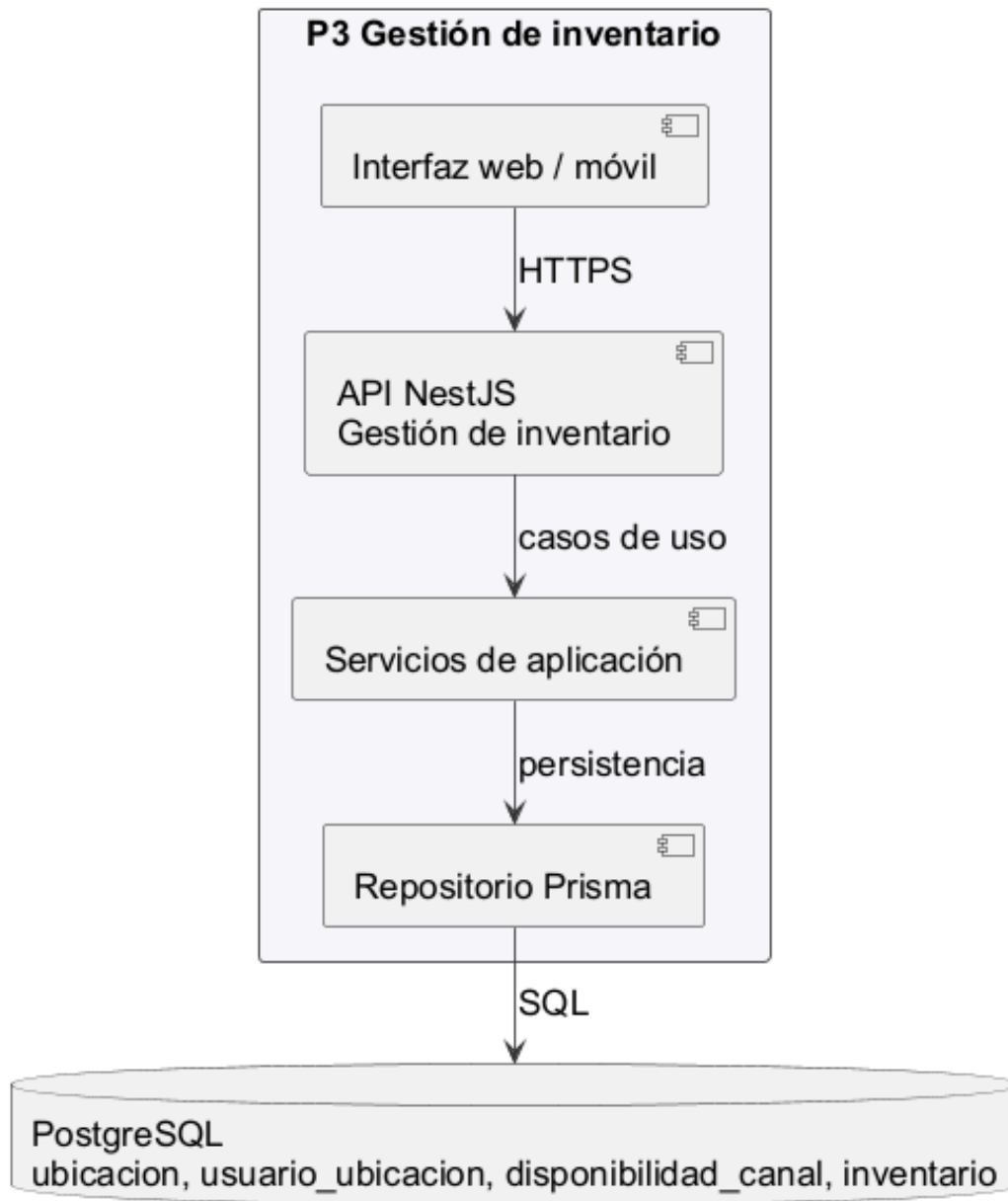
Figura 131. Componentes previstos del paquete P3
