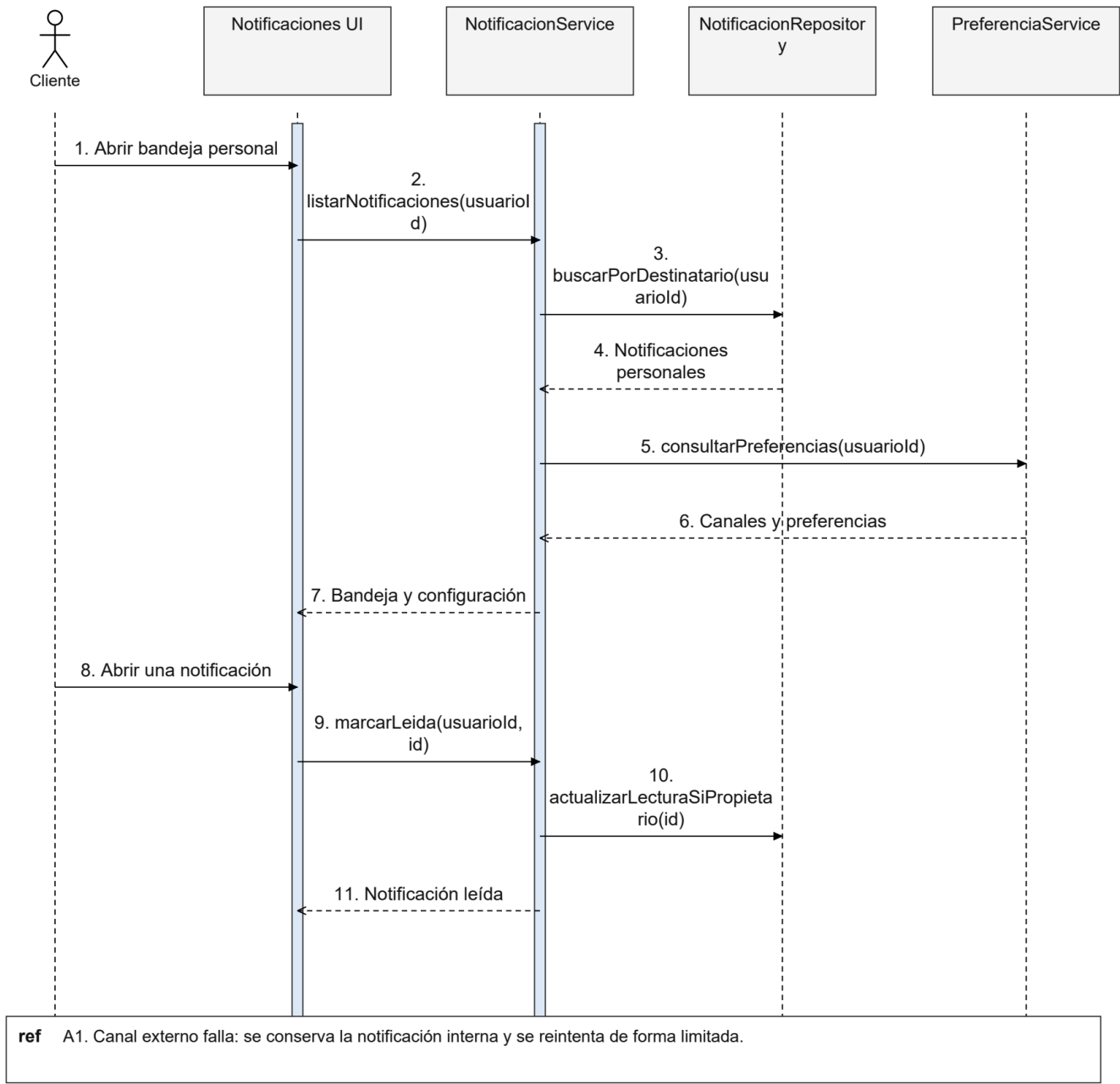
Figura 112. CU21 Secuencia de diseño
