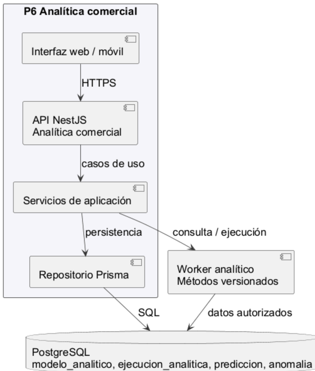
Figura 134. Componentes previstos del paquete P6
