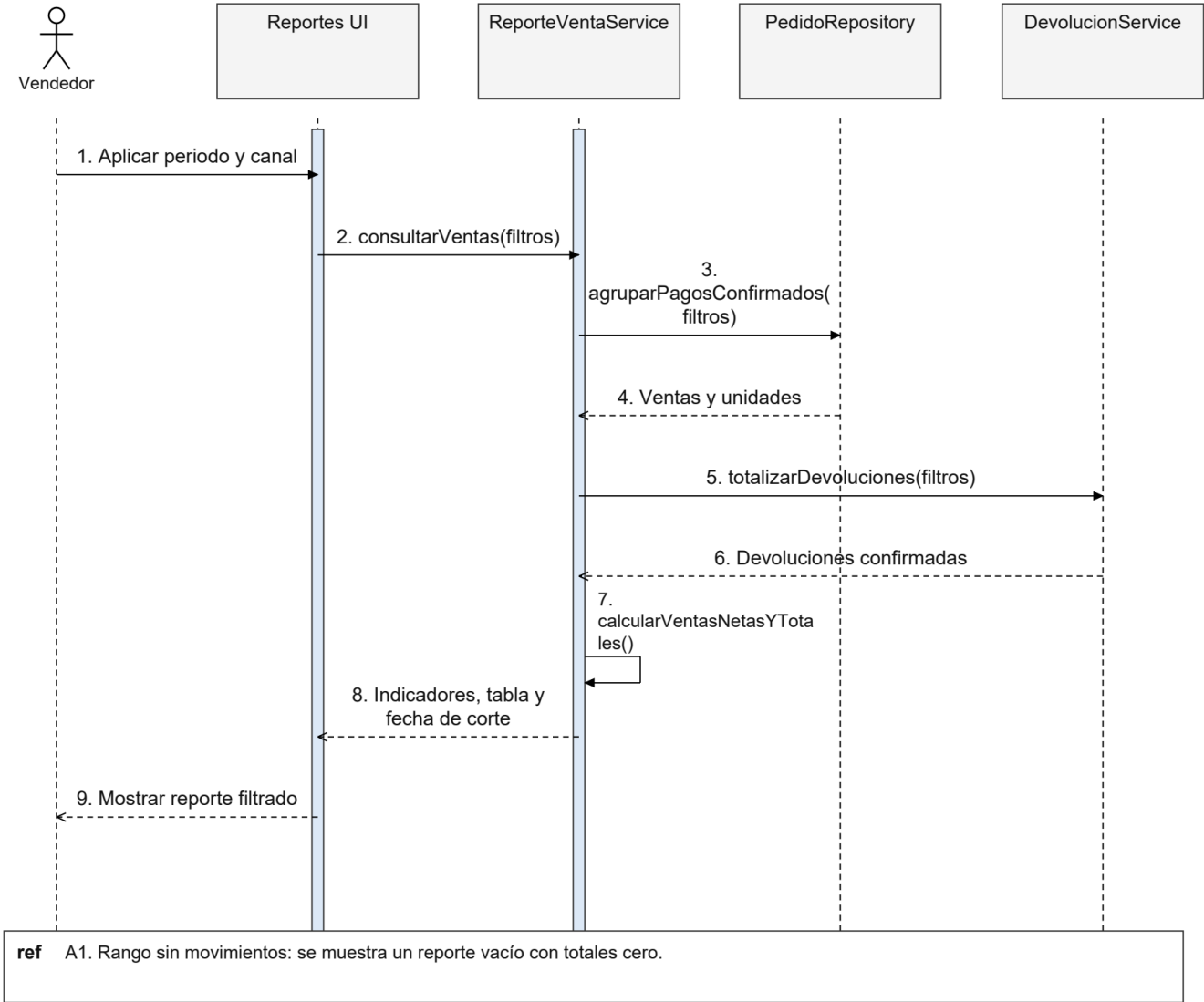
Figura 107. CU10 Secuencia de diseño
