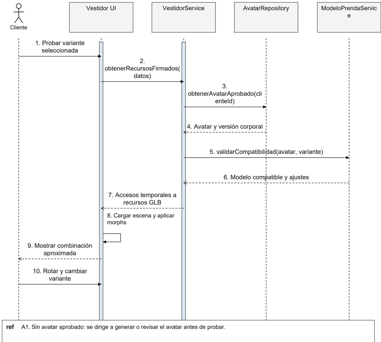
Figura 101. CU16 Secuencia de diseño
