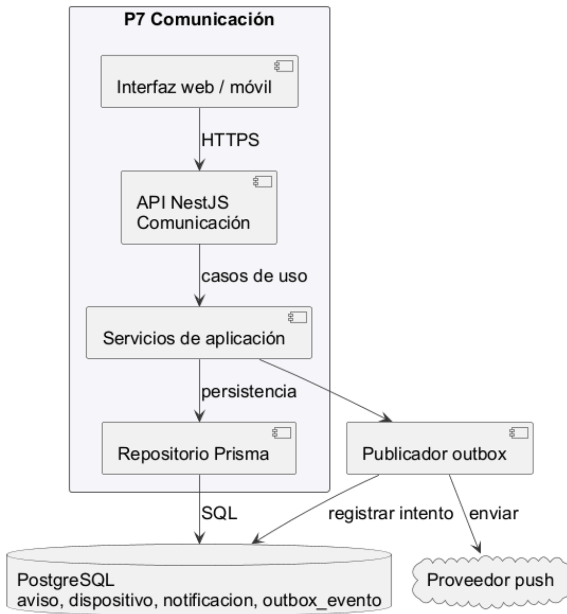
Figura 135. Componentes previstos del paquete P7
