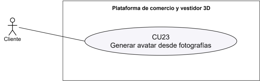
Figura 10. CU23 Actores y caso de uso
