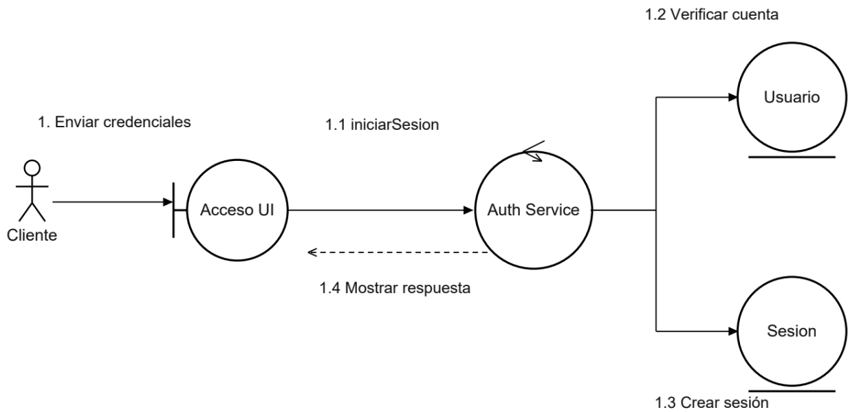
Figura 41. CU02 Diagrama de comunicación
