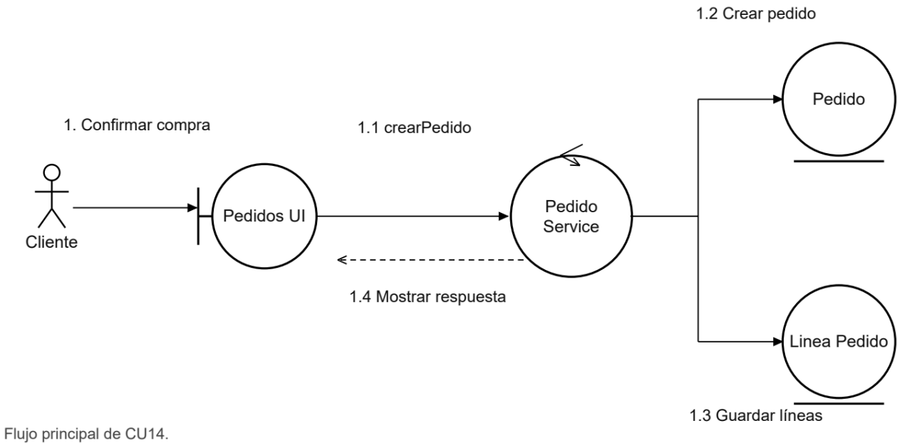
Figura 73. CU14 Diagrama de comunicación
