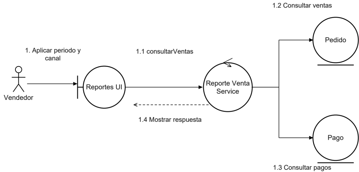
Figura 65. CU10 Diagrama de comunicación
