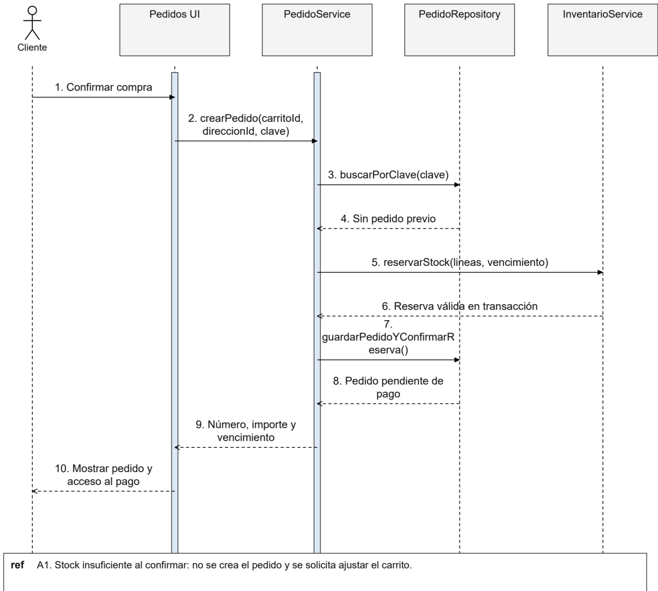
Figura 111. CU14 Secuencia de diseño
