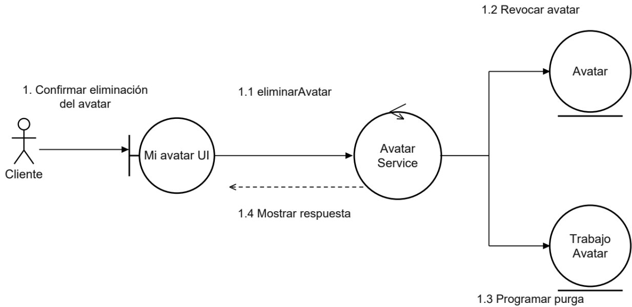
Figura 59. CU25 Diagrama de comunicación
