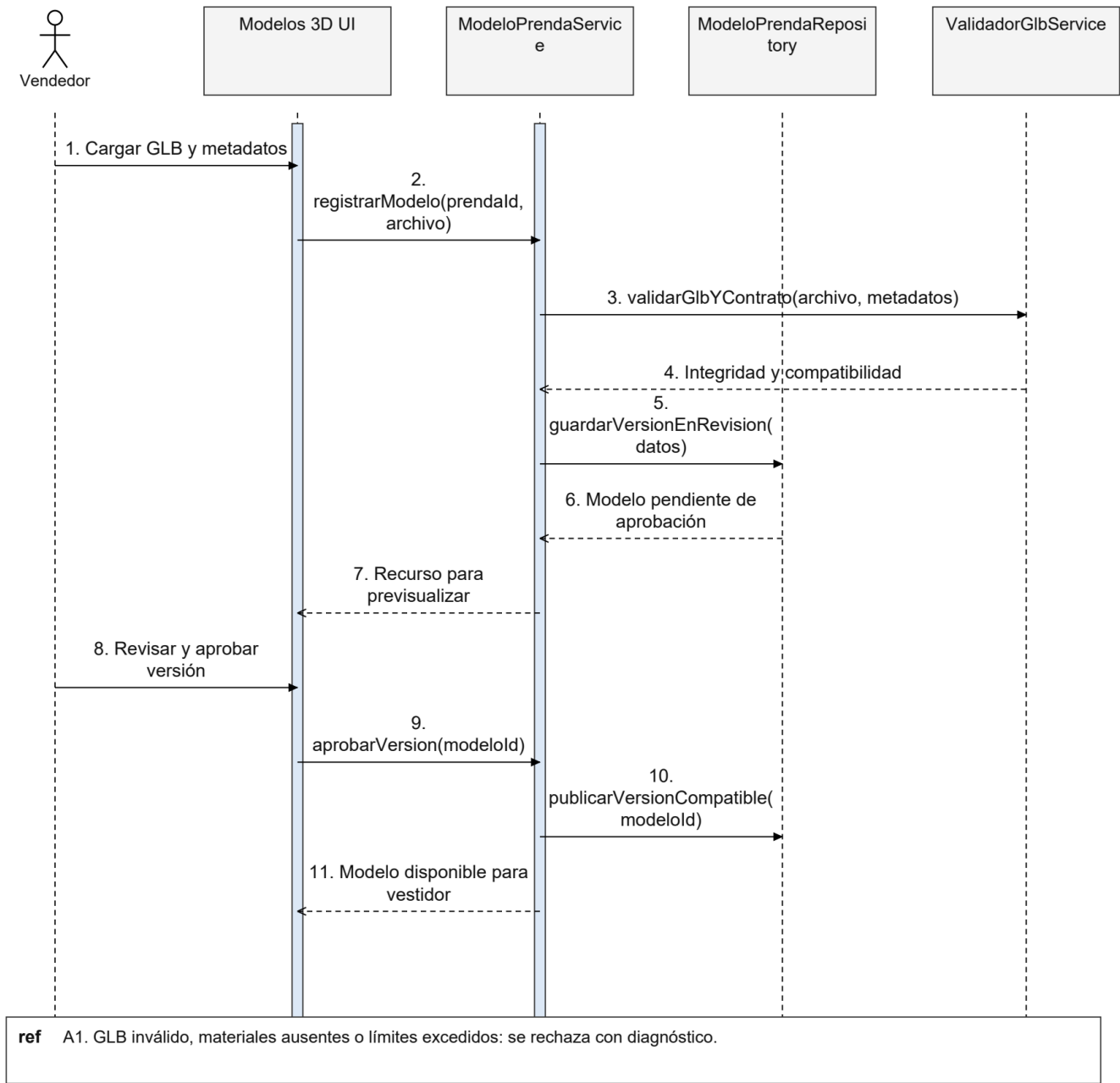
Figura 103. CU24 Secuencia de diseño
