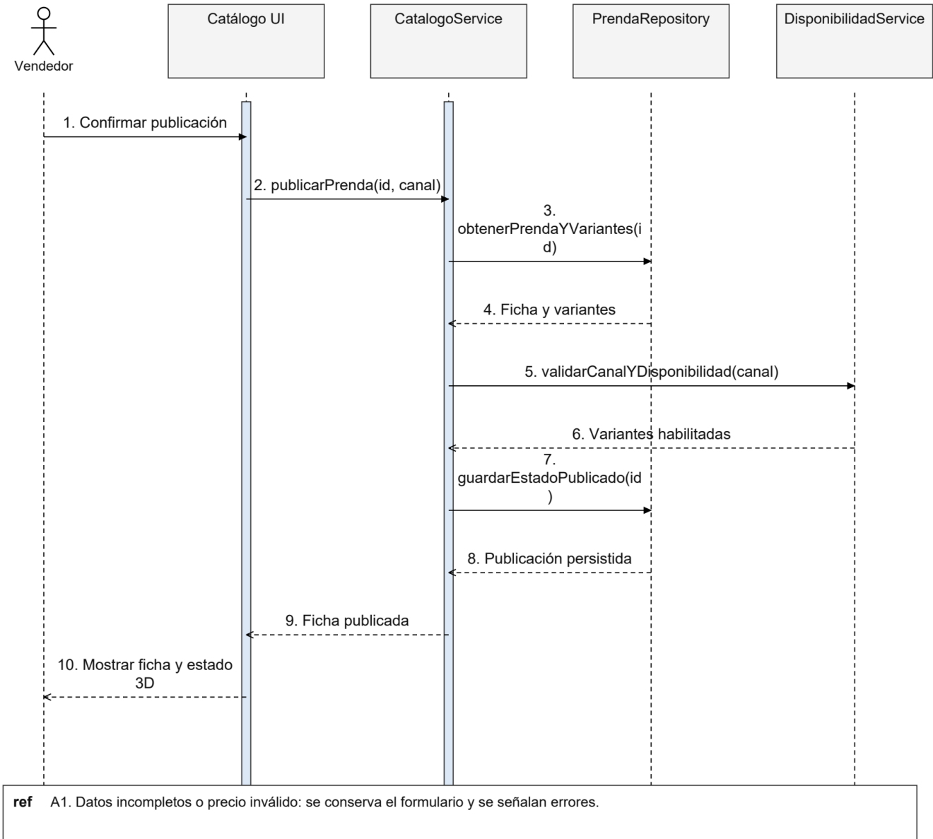
Figura 97. CU04 Secuencia de diseño
