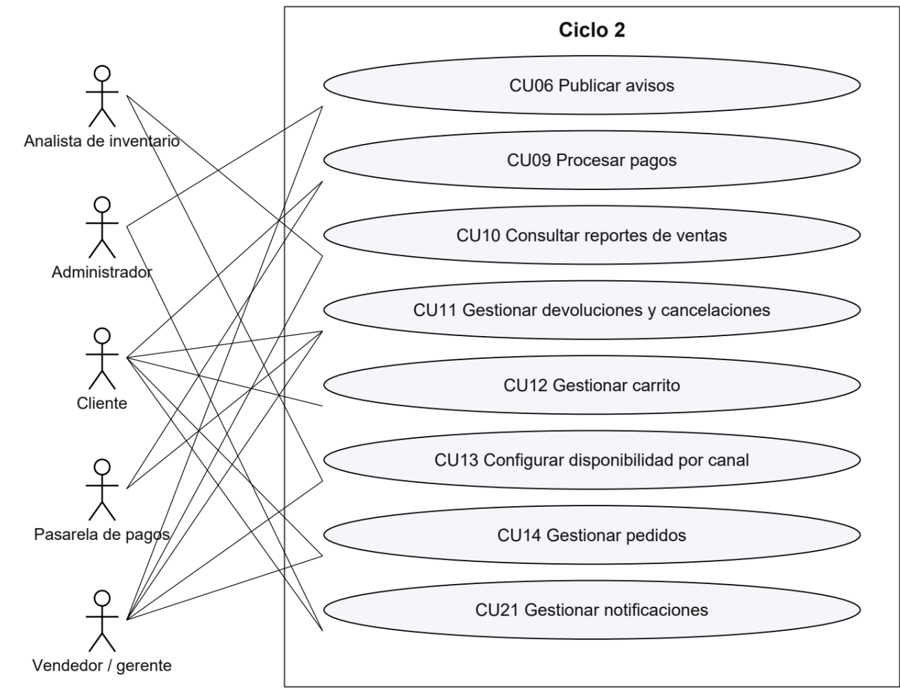
Figura 28. Asociaciones de actores y casos del ciclo 2
