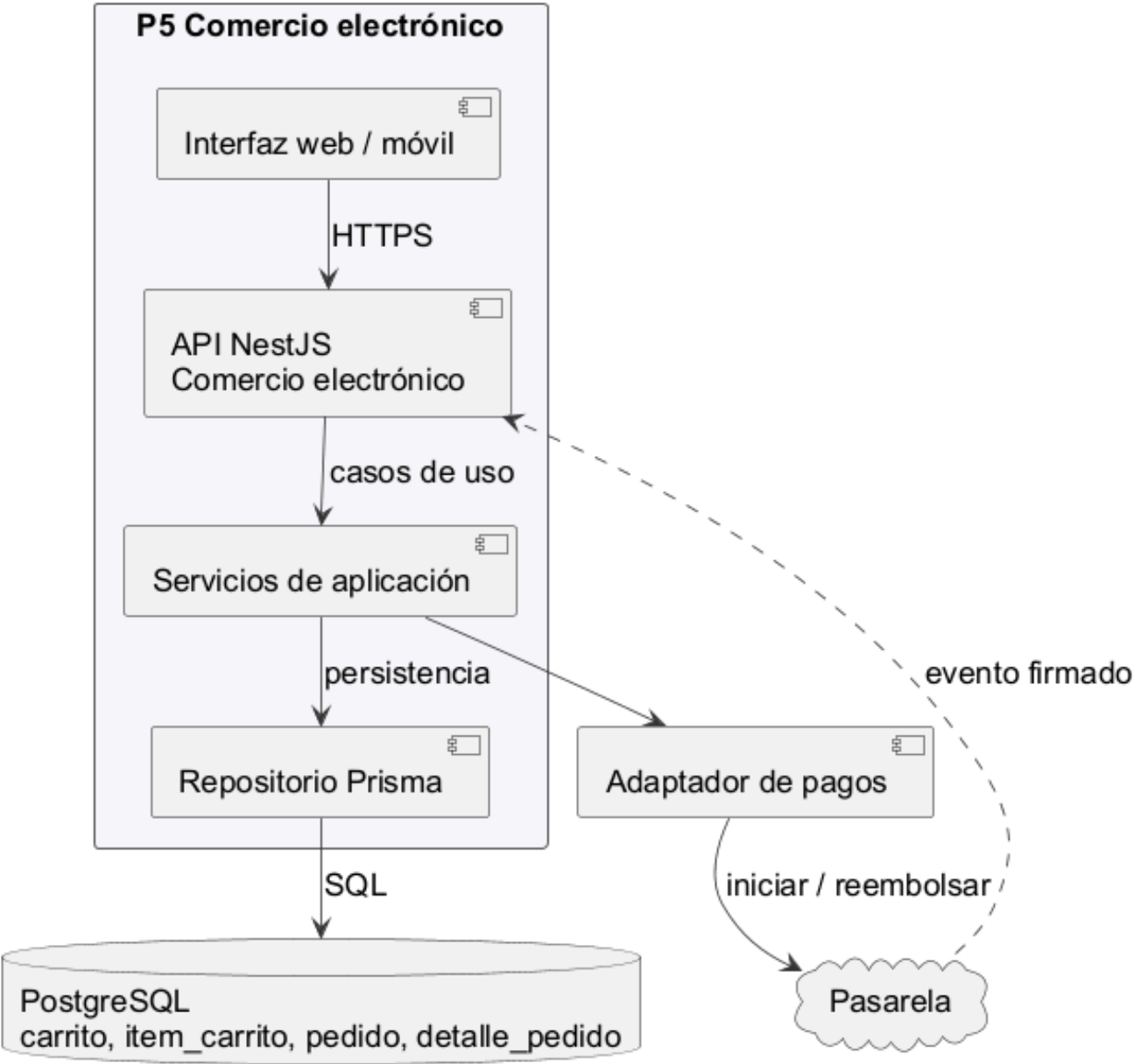
Figura 133. Componentes previstos del paquete P5
