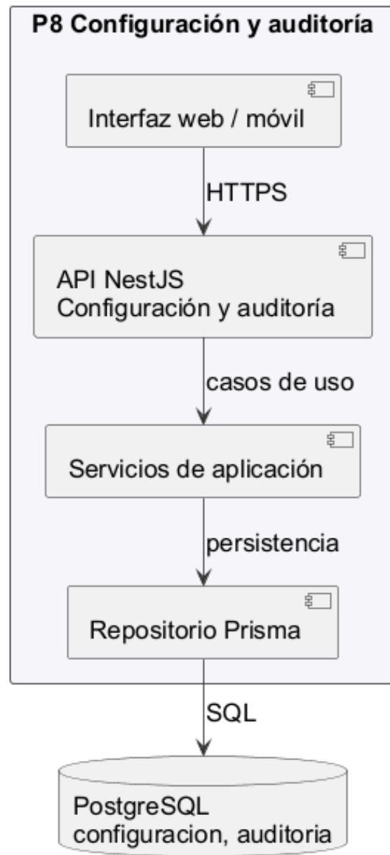
Figura 136. Componentes previstos del paquete P8
