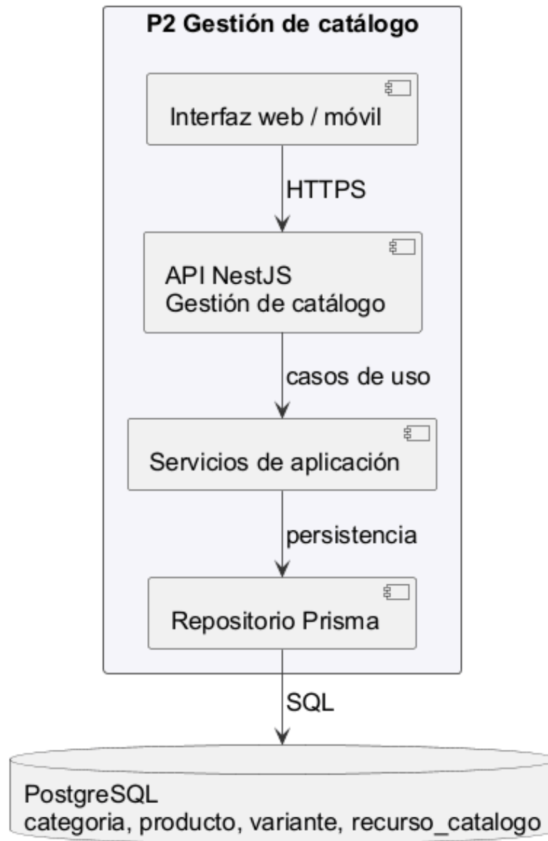
Figura 130. Componentes previstos del paquete P2
