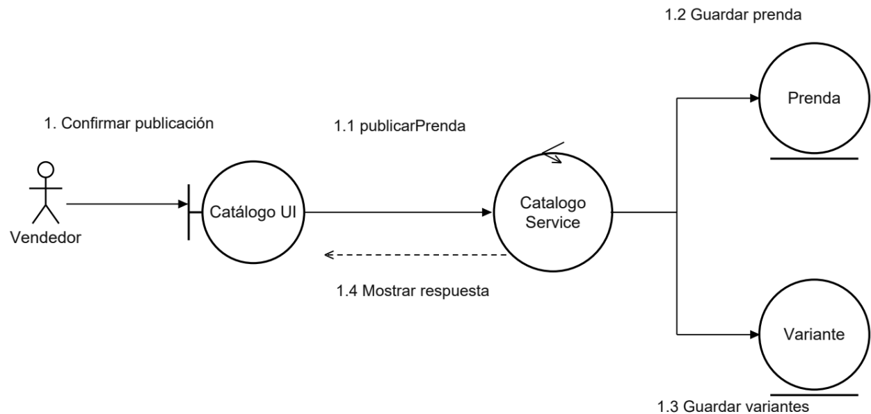
Flujo principal de CU04.
