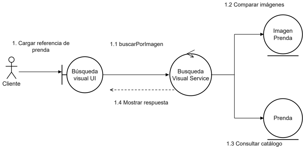
Figura 81. CU18 Diagrama de comunicación
