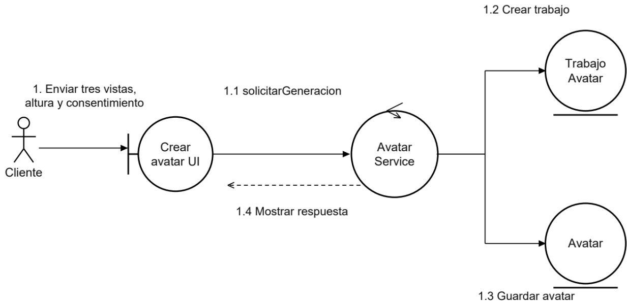
Flujo principal de CU23.
