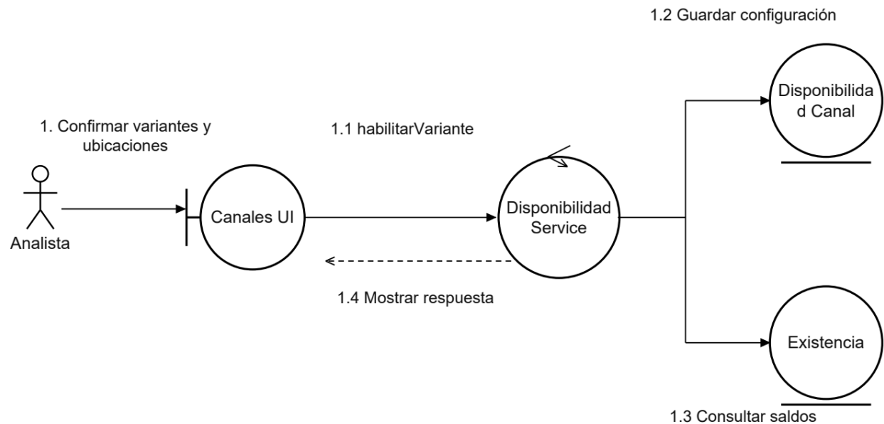
Figura 71. CU13 Diagrama de comunicación
