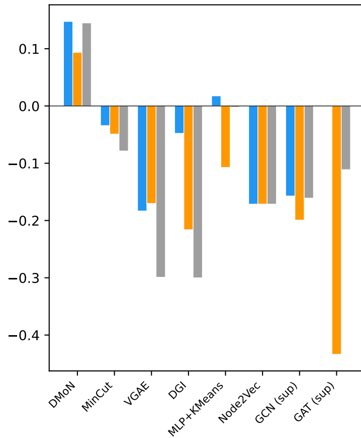
GRN
