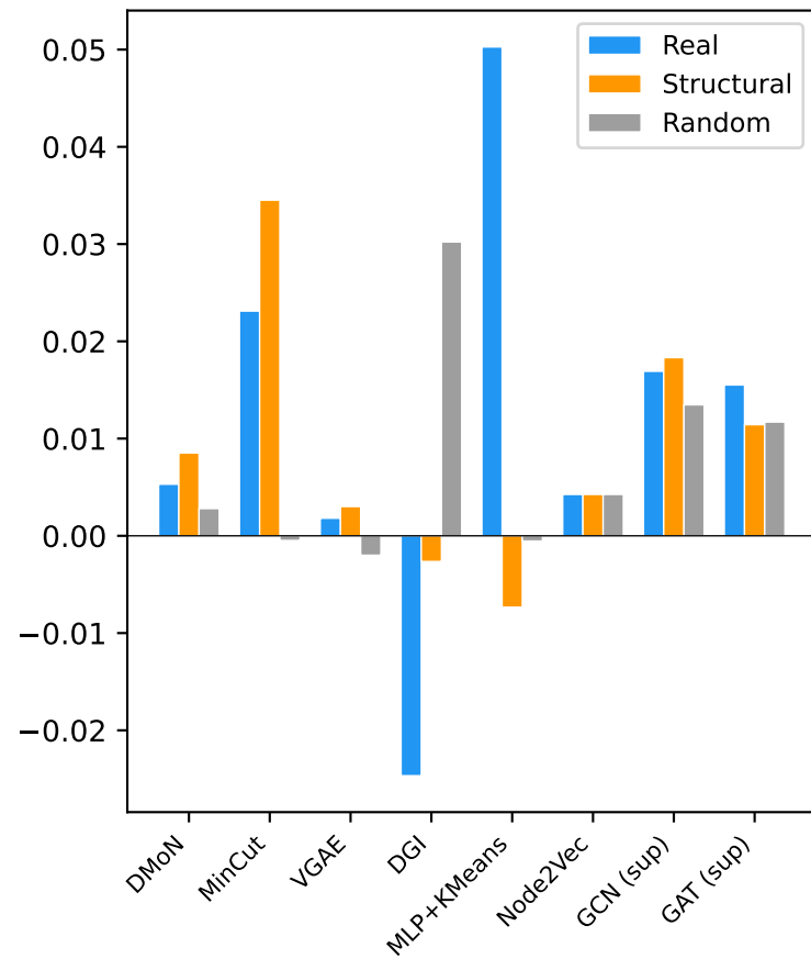
GTEx
