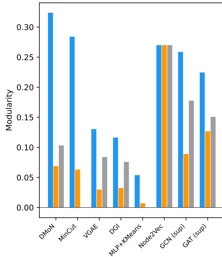
SIGNOR
