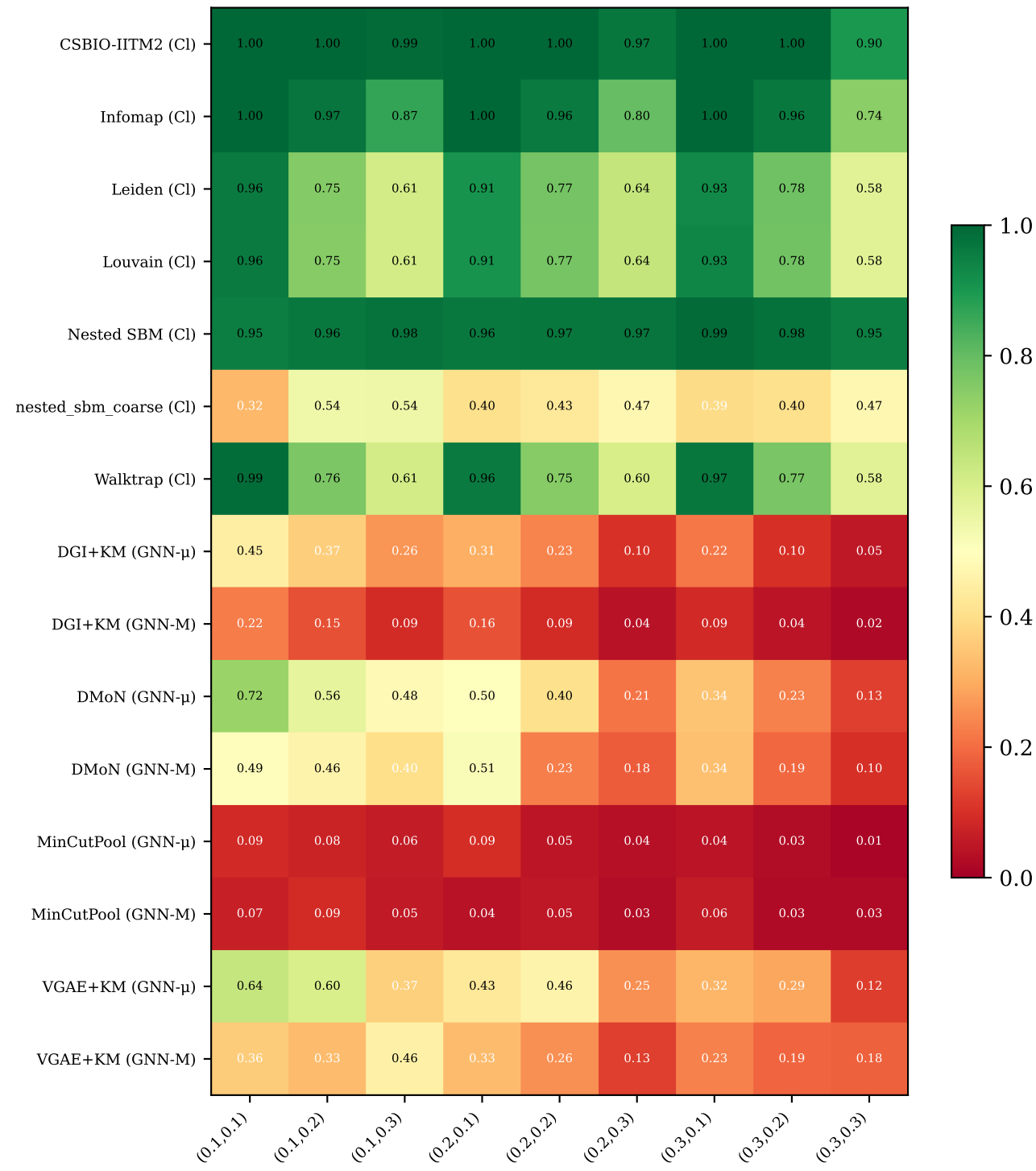
(a) Micro-level AMI
