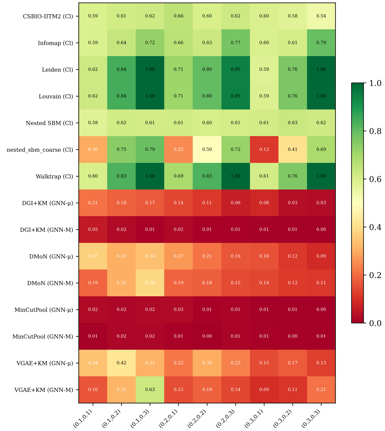
(b) Macro-level AMI
