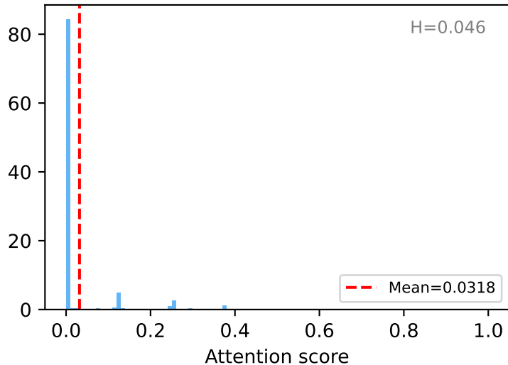
GRN
