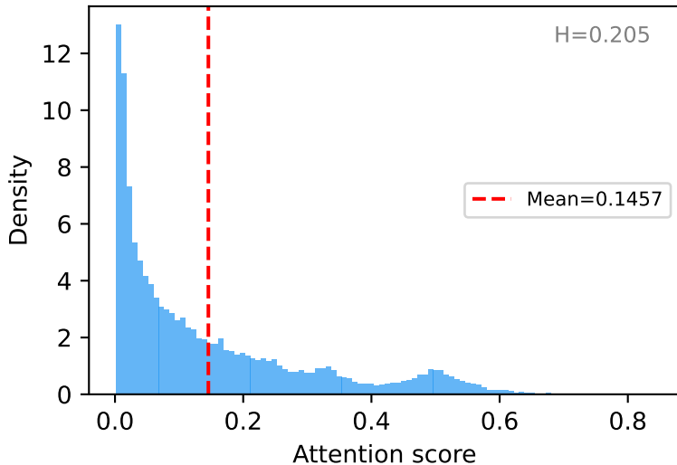
SIGNOR
