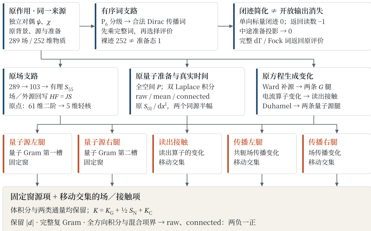
图 1 同一原作用，两份证词；五项缺一不可。 上支路保留词序、分级和评价方式；下支路将原物质反馈、原场回写与量子准备读数相接。两条量子源腿含 Duhamel 变化，使用固定窗；两条场传播腿与读出接触项使用随外动量移动的双球交集；朱红标出的五项缺一不可。窗口标注对应本案零输出动量、两窗等半径的设置，一般窗口分配见第 7.4 节。箭头表示依赖，不表示数值相等。
