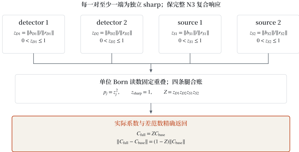
图 6 四个 Born 重叠直接生成实际 Coulomb 修饰。 D1 / D2 是 detector 左右腿, S1 / S2 是 source 左右腿。各 b_j 为原底层响应, r_j 为完整 N3 响应, p_j = z_j^2 是单位态的 (3,0) Born 值。每一对至少有一端为独立 sharp, 完整规范分子才能精确返回底层; 两个完整范数仍保留。四个正重叠之积给 (13.8) 的实际系数及差范数, 并进入同一个 whole289 Newton 包。
