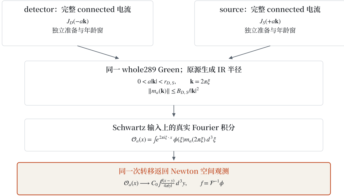
图 5 两个实际端点共享同一次 Fourier 转移。两个 created N2 connected 电流分别取 J_D(-ak) 与 J_S(ak) ，各保自己的准备和年龄窗。图中 m_a 是 (12.11) 的完整两端收缩， C_0 = L(0, S_0) ；共同 IR 半径与预算由实际连续性及全方向 Green 自产，窗外按原定义置零。Schwartz 输入支付同一次真实积分， f = \mathcal{F}^{-1}\phi ，只出现一次 4\pi 。该 raw connected 读口使用 (12.9) 的原归一，不增一个 hc_b 分母。
