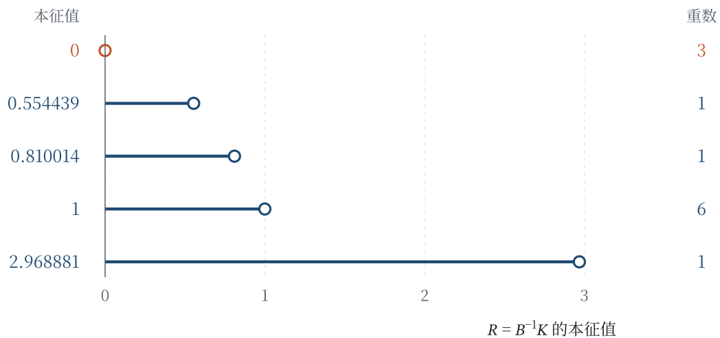
附图 A3 native P286 标量—规范裸二次块。 左列为 R = B^{-1}K 的本征值, B 为原生实标量配对, 右列为重数; 12 个方向中 3 个为零 (朱红), 9 个为正, 三枚非有理本征值是 (A.5) 三次式的根, 按有理隔离区间的小数显示。零空间与稳定子切向对应; 完整耦合传播另外见 §4。
