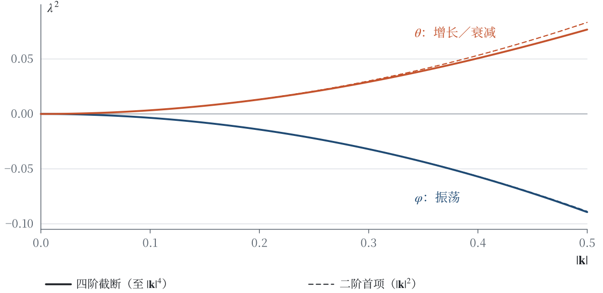
图 2 原时间中的两条软支。 实线为 (5.10)–(5.11) 在 \mathbf{k} = 0 附近的四阶截断，虚线为二阶首项，横轴展示 0 \leq |\mathbf{k}| \leq 0.5 ，渐近余项为 O(|\mathbf{k}|^6) 。纵轴为原时间增长变量 \lambda^2 ：零线以下是振荡支 \varphi （深蓝），以上是增长/衰减支 \theta （朱红）；后者的四阶项在所示范围内已与首项分开。截断式不是有限动量的精确色散式。
