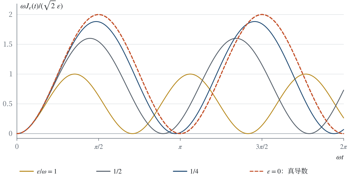
图 3 有限电流如何趋向真导数。 实曲线采用 (8.14) 的 \epsilon/\omega = 1, 1/2, 1/4 (金、灰、深蓝), 朱红虚线为归一化真导数 1 - \cos 2\omega t , \omega = 18\sqrt{15}/125 。横轴 \omega t 使用原时间, 不是固有时。纵轴为单位占据态的 \omega J_\epsilon/(s\epsilon) ; 原有幅度场的电流乘四。有限幅度既改变振幅, 也改变振荡频率。
