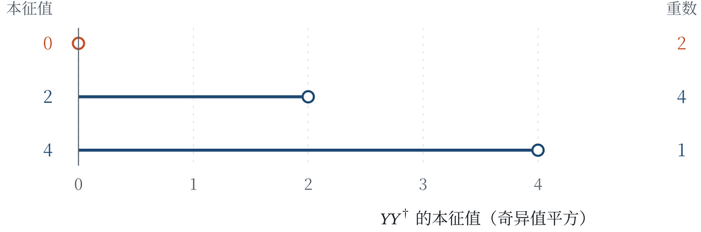
附图 A2 联合真空的非零奇异值与核。 左列为 YY^\dagger 的本征值 (奇异值平方), 右列为重数; 朱红的零本征值 (重数 2) 给出 \text{rank } Y = 5 。来自完整 7 \times 21 楔映射的 Gram 矩阵; 图中裸奇异值的身份区别于 §6 的原频率谱。
