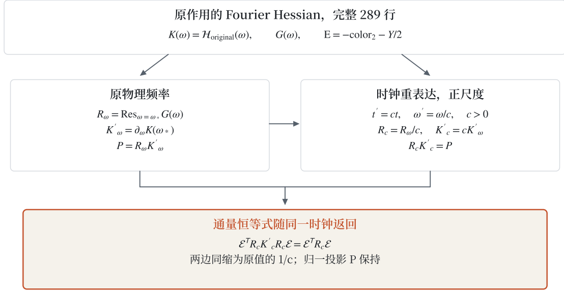
图 4 同一原作用下的时钟重表达。固定原 source 支、单位空间方向及已生成简单极点范围, t' = ct 的正尺度重表达使 R_c = R_{\omega}/c 、 K'_c = cK'_{\omega} 。图中的 \mathcal{E} 是字面 E 插入四个规范槽得到的完整 289 维映射; 实际混合输出先保留, 再收缩。归一投影与通量恒等式保持, 两端张量共同缩为原值的 1/c , 对应 (11.9)–(11.11)。
