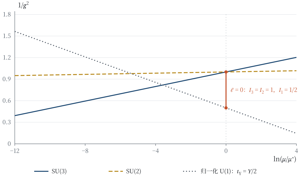
附图 A1 指定库存的三条仿射读数。 横轴为库存跑动坐标 \ln(\mu/\mu^*) , 不是原时间; \ell = \ln(\mu/\mu^*)/(8\pi^2) , 三条线即 (A.2), 取原生 \sigma = 1/2 , 未引入阈值、实验拟合或 GeV 标定。朱红竖段标出 \ell = 0 处 I_3 = I_2 = 1 而 I_1 = 1/2 的缺口。
