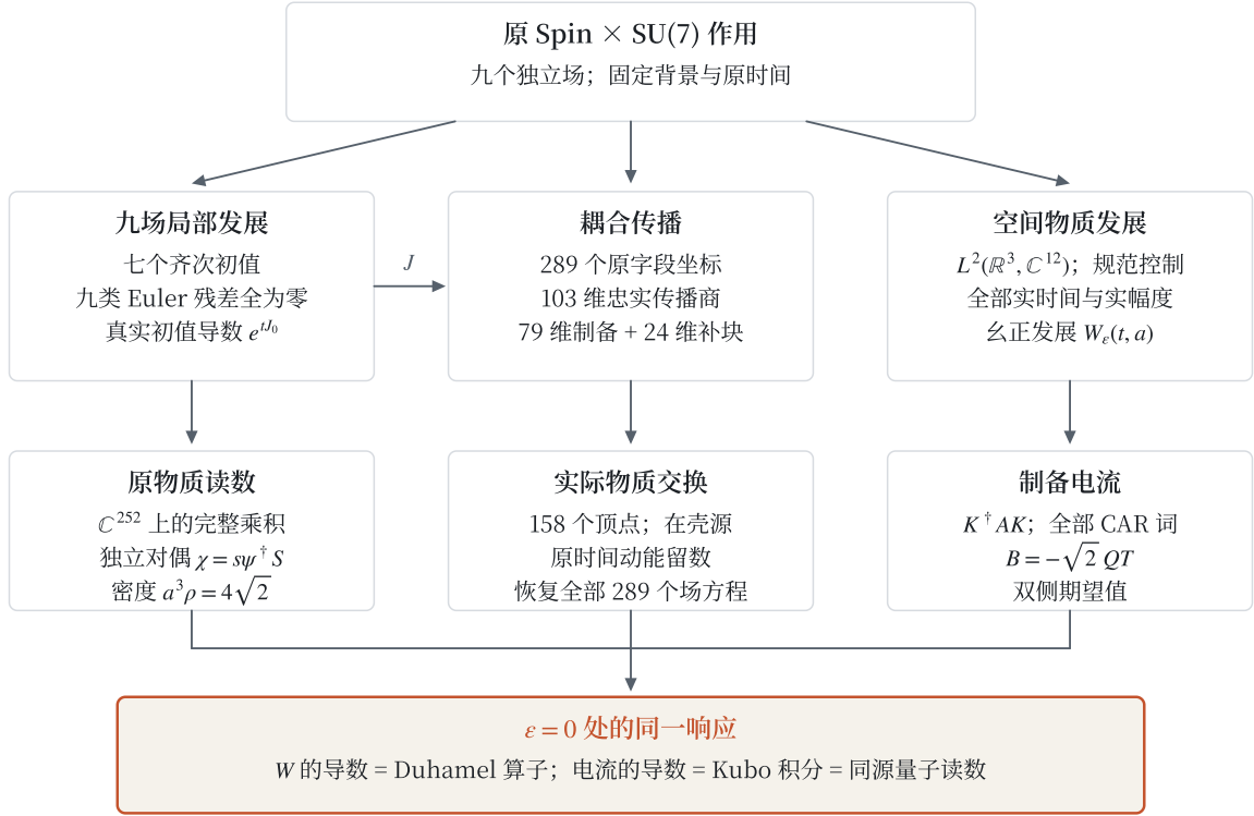
图 1 同一电流的来路与返回。 左、中两列从原作用生成九场发展和受约束传播，右列从原物质作用生成空间准备与有限发展。朱红底框是三条路径的汇合处：作用电流、双侧变分及 Kubo 积分在 \epsilon = 0 处给出同一响应。箭头携带显式的场、方程或源映射，不把三个域等同；原字段恢复箭头表示实际方程恒等式，而非只保留某个行列式。三条发展路径的输入分别见上表。
