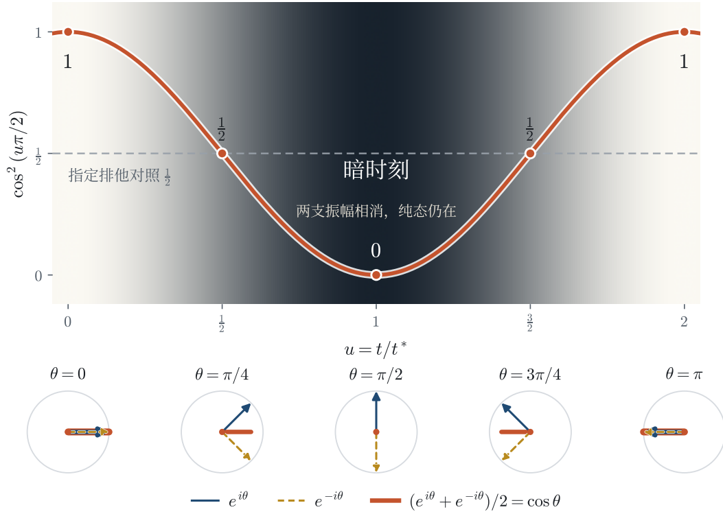
图 5 | 五个刻度上的相干读数。 例 1.1(c) 的五个数, 在这里连成一条会变暗的曲线。横轴 u = t/t^* , t^* = \pi/(2\omega) 。实线为 \cos^2(u\pi/2) , 虚线为指定排他对照的常值 1/2 ; 五个标记点依次为 1, 1/2, 0, 1/2, 1 。底色随同一读数 \cos^2(u\pi/2) 线性变亮, 暗时刻因此在画面上就是暗的; 它是曲线的第二种编码, 不是另一组数据。下方五个圆与五个标记点同列对齐, 画上、下两条单位相位振幅 e^{\pm i\theta} 及其平均 (e^{i\theta} + e^{-i\theta})/2 = \cos \theta (朱红短杆), 短杆长度的平方即上方读数; 箭头本身不是概率。暗点 u = 1 表示指定效应中的相消, 不表示态失去相干。曲线由解析式直接求值, 既不是实验散点, 也不含频率拟合。
