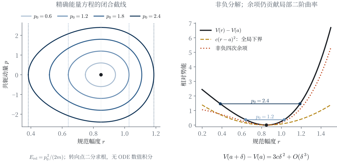
图 4 | 等能轨道与强制能量控制。 理论公式的数值可视化。左：四个指定初始冲量的能量截线 p = \pm\sqrt{2m(E_{\text{rel}} - [V(r) - V(a)])} ，其中 E_{\text{rel}} = p_0^2/(2m) ；转向点通过单调两支上的二分求根得到，正负动量分支在 p = 0 处闭合； p_0 = 1.2 与 p_0 = 2.4 的转向半径以同色竖直线标出。这里没有以数值 ODE 积分替代全时存在证明。右：完整势差、全局二次下界 c(r-a)^2 和非负余项 3(r-a)^2(r+a)^2/(4\sigma N) ；两条水平细线是同一对 p_0 的相对能量，与势差曲线的交点正是左图同色点线所示的转向点；余项近 r = a 仍为二阶。全部参数来自表 A2，没有拟合数据。
