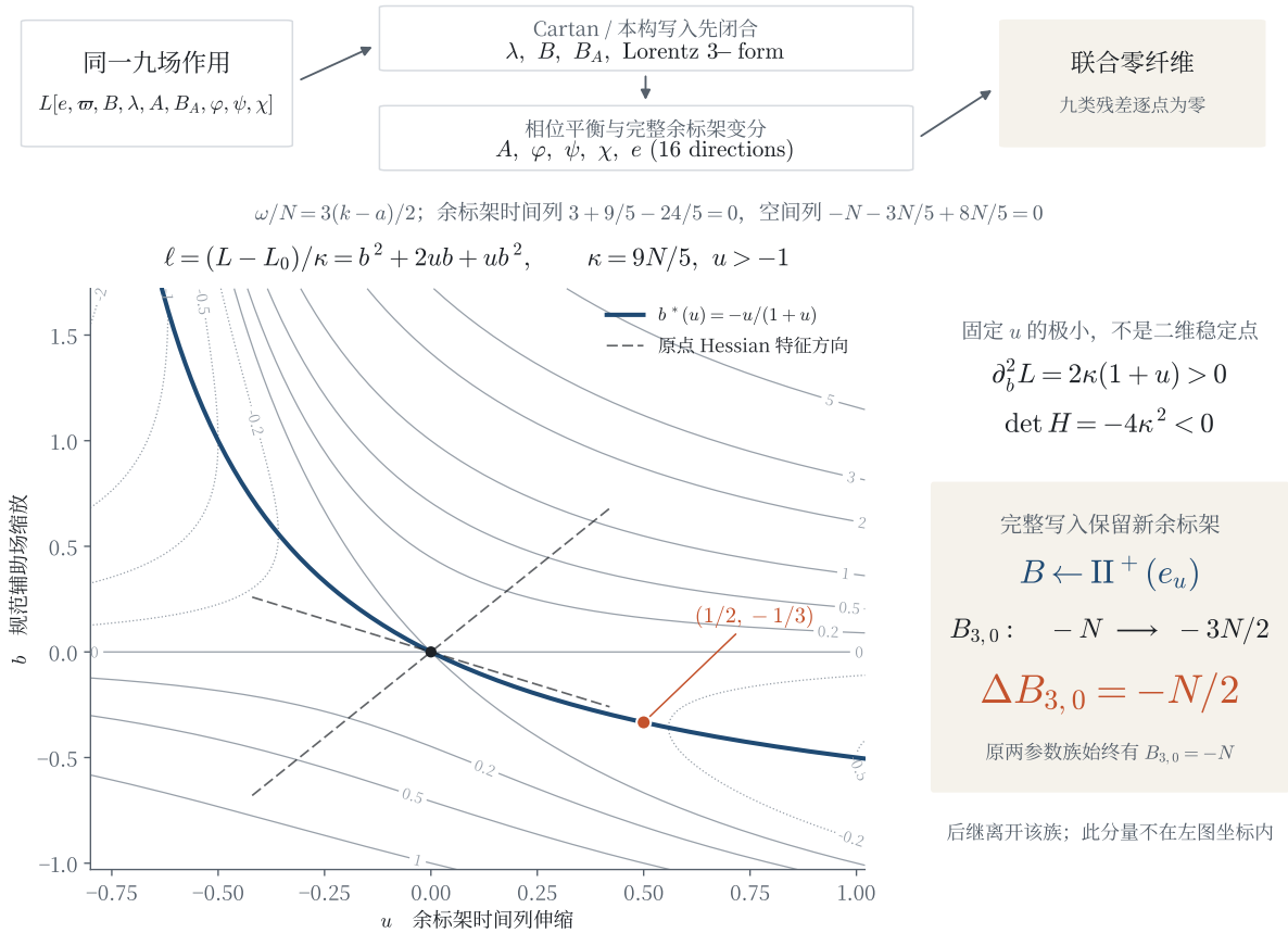
图 2 | 混合密度与截面外的后继。 上部为九场构造依赖示意；下部等高线由 \ell = (L - L_0)/\kappa = b^2 + 2ub + ub^2 直接求值。粗线 b^* = -u/(1+u) 是固定 u > -1 时的 b 向极小线，不是二维稳定平衡轨道。长虚线标出原点 Hessian 的两条特征方向；点线为负值等高线。种子点 (1/2, -1/3) 旁的独立框记录完整写入： B_{3,0} 从 -N 变为 -3N/2 ，故变化为 -N/2 。这个分量不作为 (u, b) 平面中的箭头长度或第三个轴。上部的相位式与时间/空间余标架平衡分别对应 (4.11) 与 (4.17)；下部是固定截面的密度，不是完整场空间的稳定性图。
