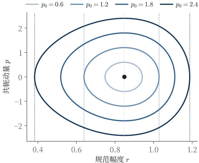
精确能量方程的闭合截线
