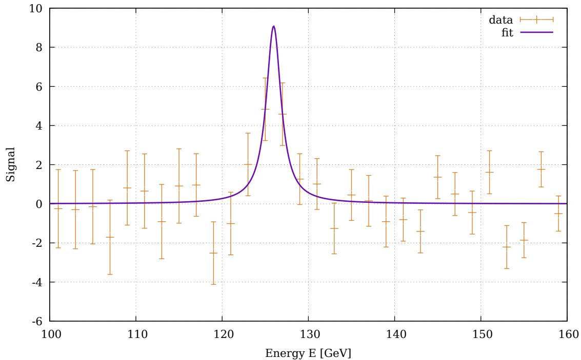
Higgs Breit-Wigner fit
