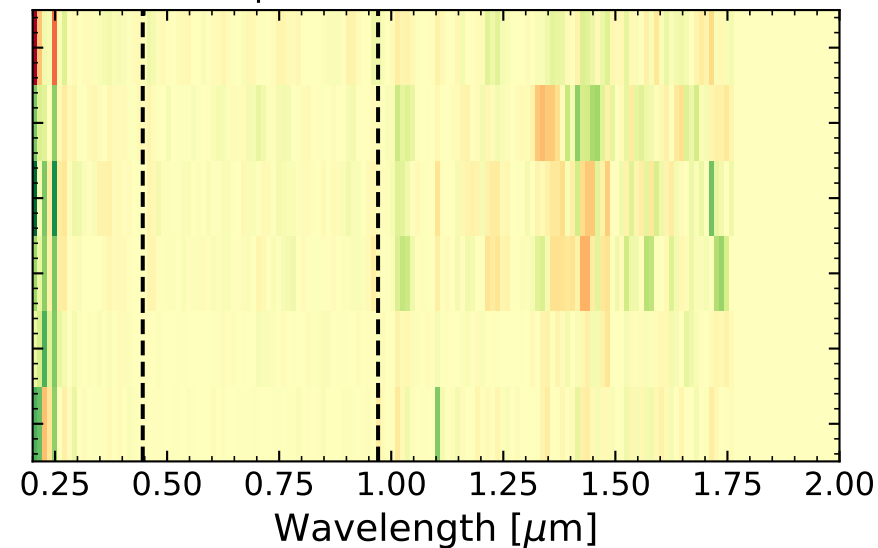
Proterozoic | HabEx/SS
