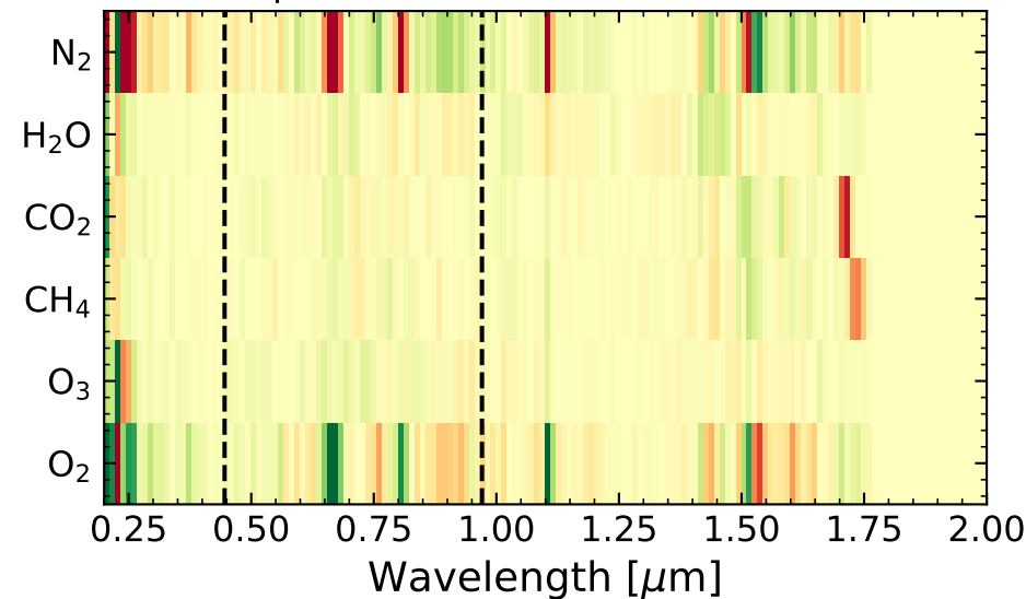
Modern | HabEx/SS
