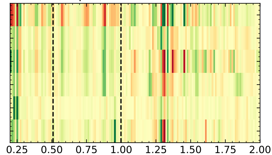
Proterozoic | HabEx/SS
