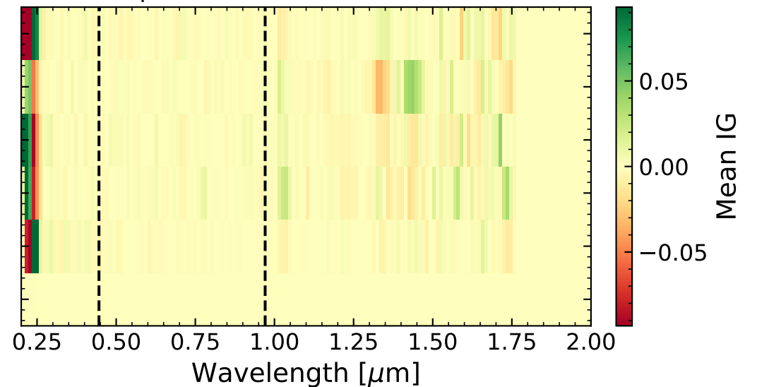
Archean | HabEx/SS
