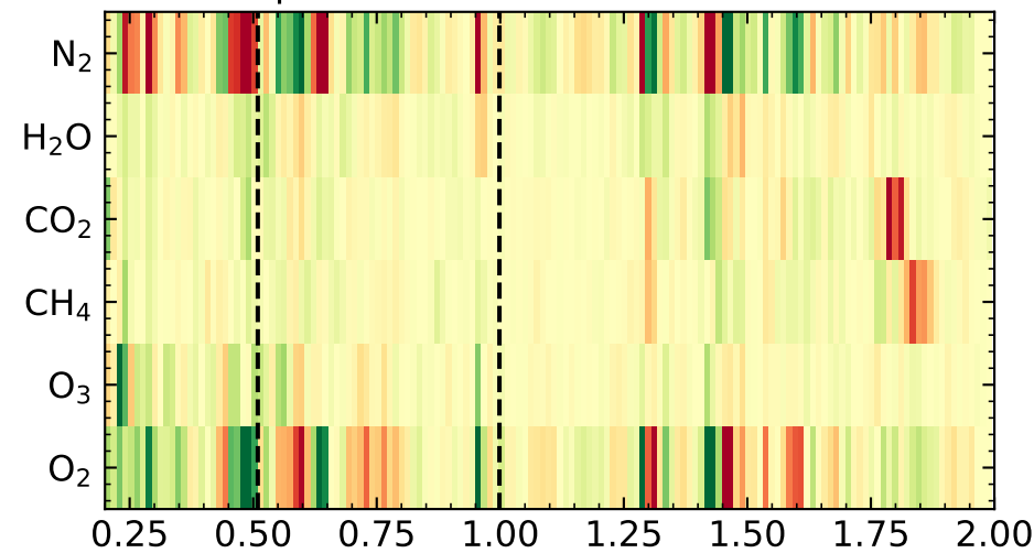
Modern | HabEx/SS
