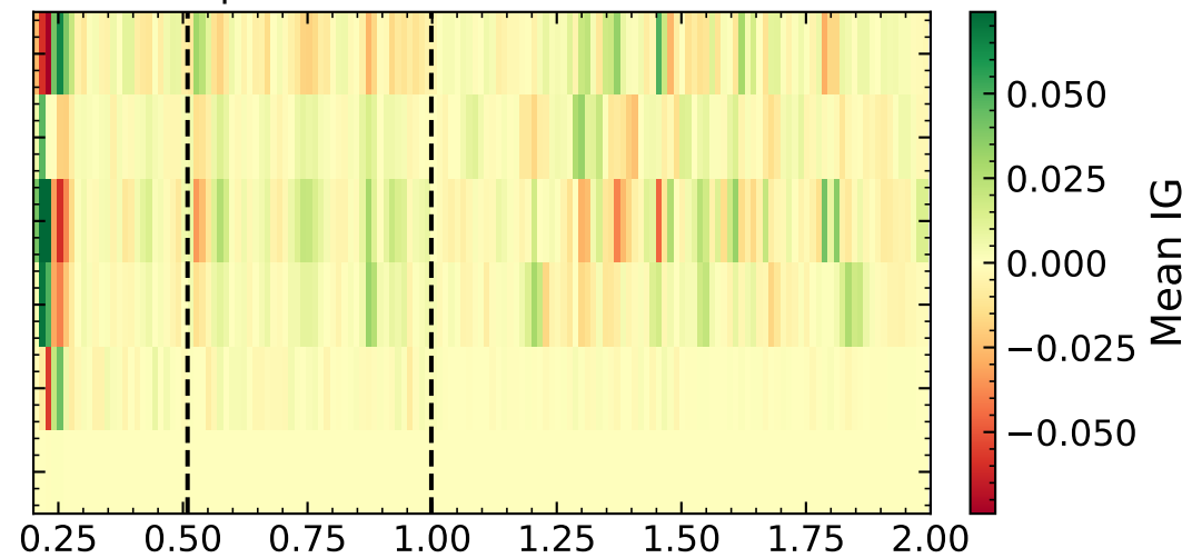
Archean | HabEx/SS
