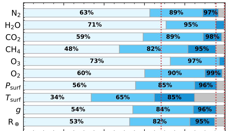
HabEx/SS - Modern
