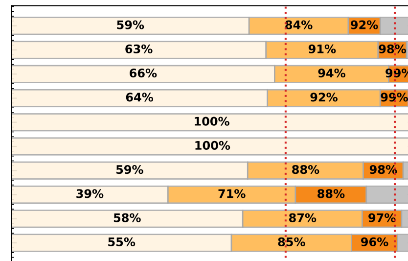
LUVOIR-B - Archean
