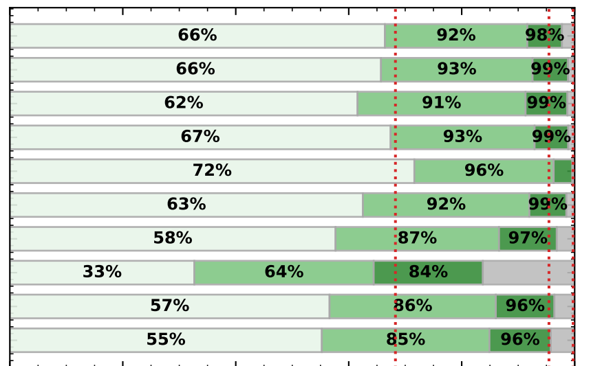
HabEx/SS - Proterozoic
