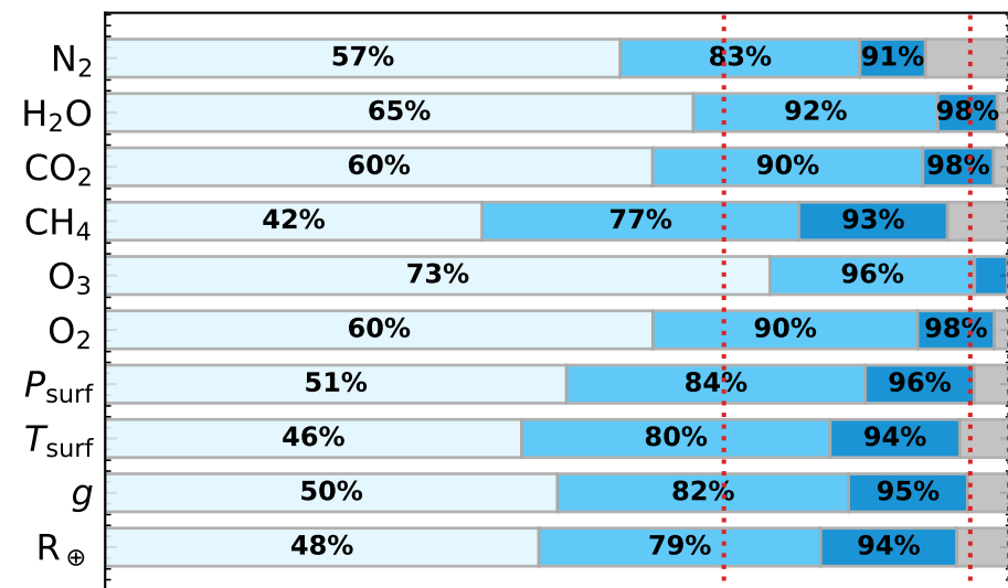
LUVOIR-B - Modern
