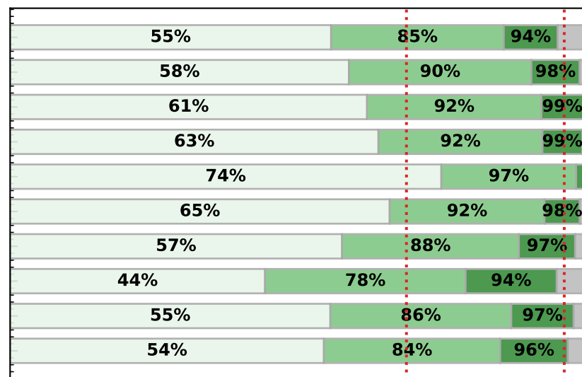
LUVOIR-B - Proterozoic
