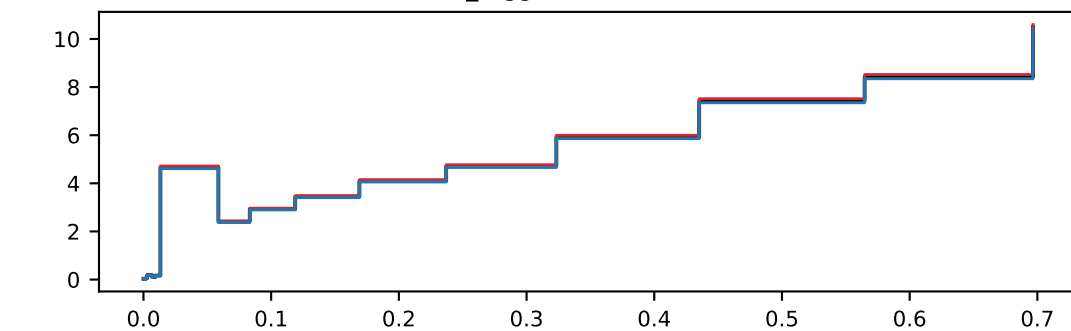
Other_Higgs (nom rate=55.09)
