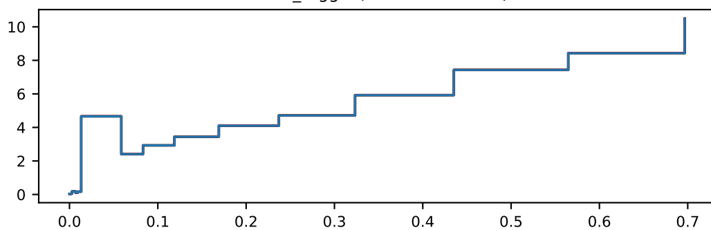
Other_Higgs (nom rate=55.09)
