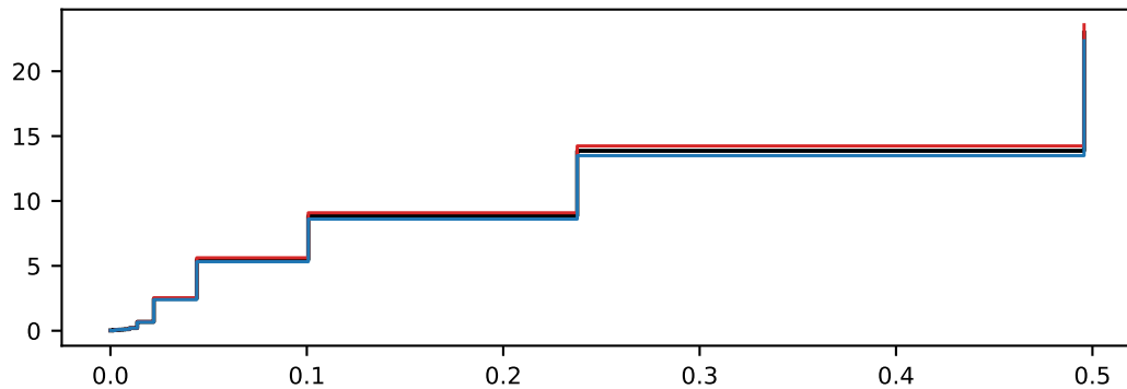
Other_Higgs (nom rate=55.28)
