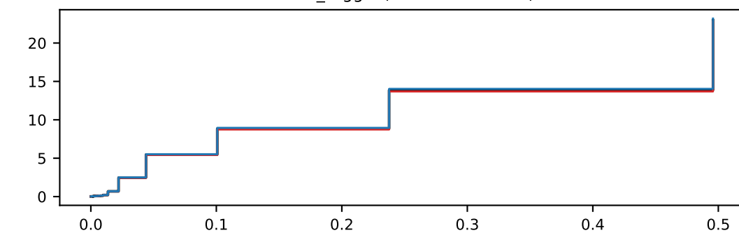
Other_Higgs (nom rate=55.28)
