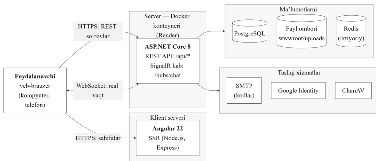
2.1-rasm. Tizimning umumiy arxitekturası va joylashtırish sxeması
