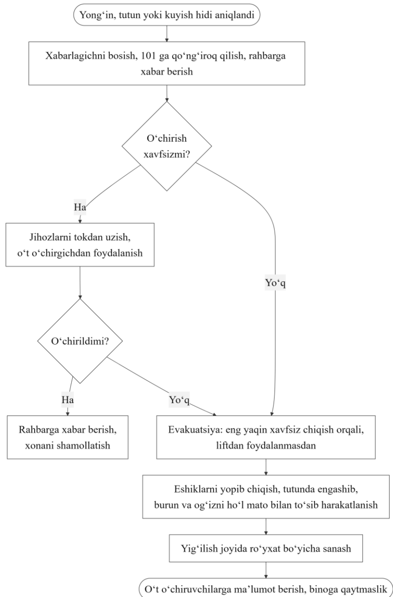
4.4-rasm. Yong'in sodir bo'lganda xodimlarning harakatlar algoritmi
