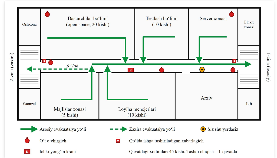
IT-ofis qavatining evakuatsiya reja-sxemasi
