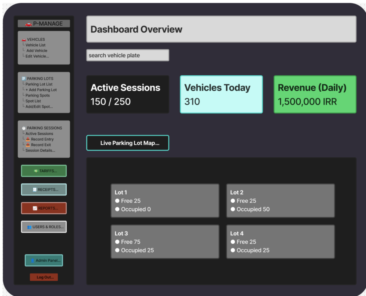
Navigation Design رسم با نرم افزار فیگما
