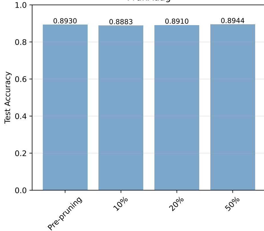
PrunAdag
