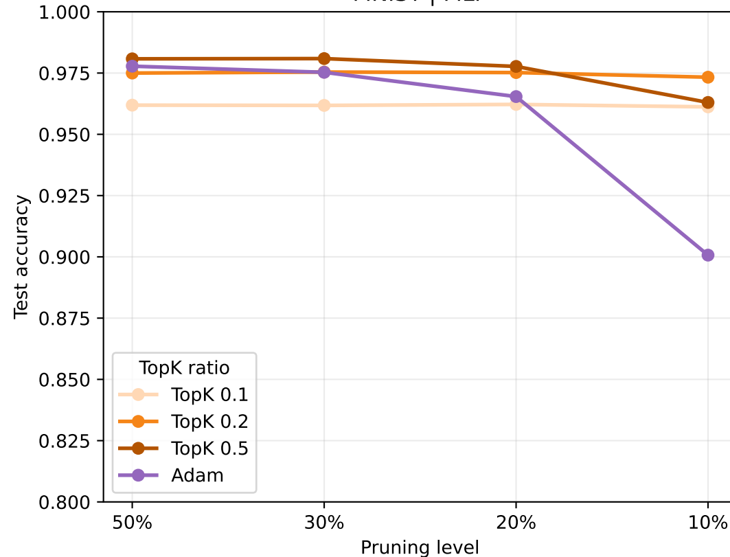
MNIST | MLP
