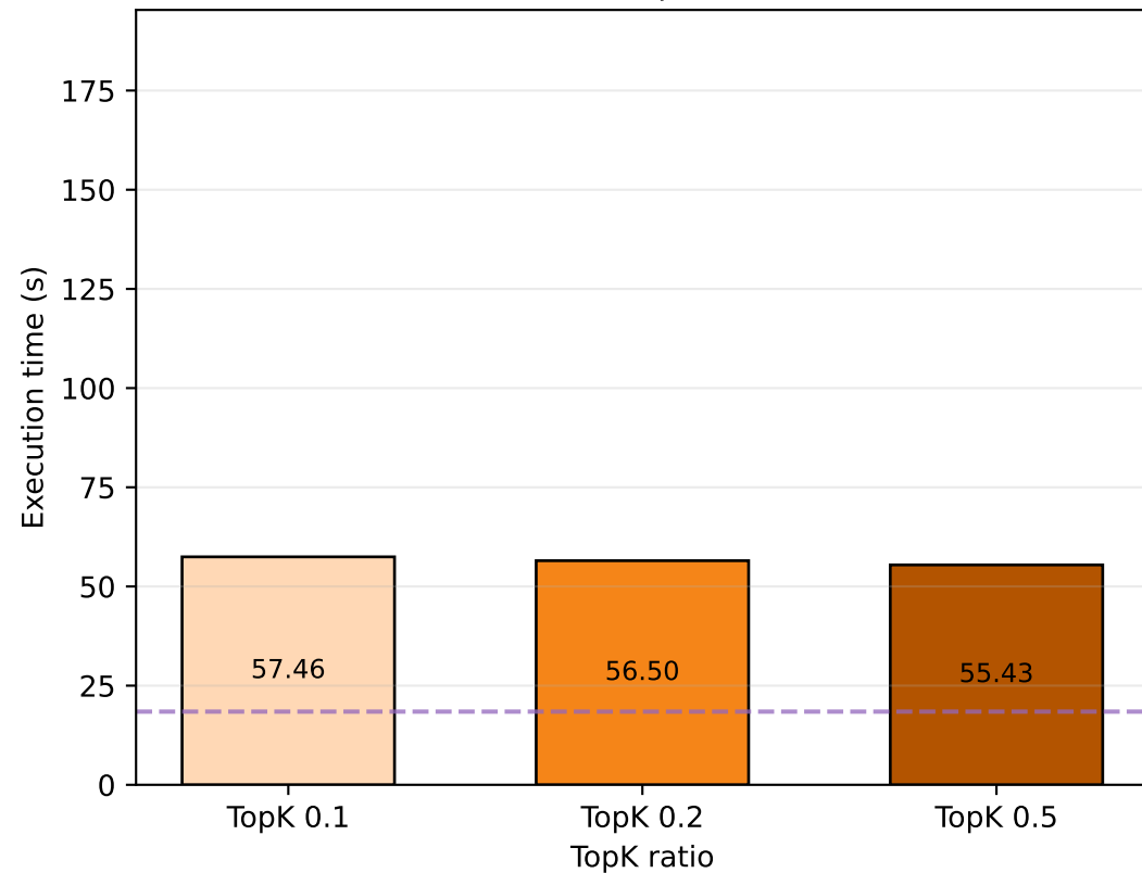
MNIST | MLP
