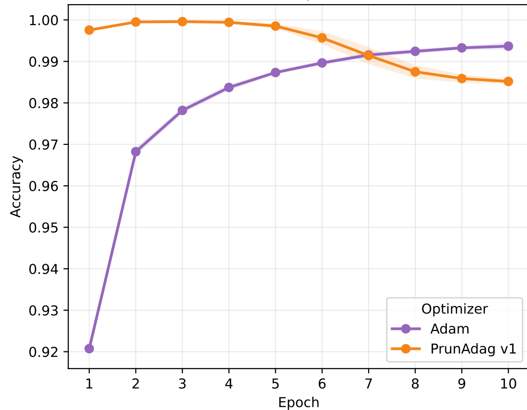
MNIST | MLP
