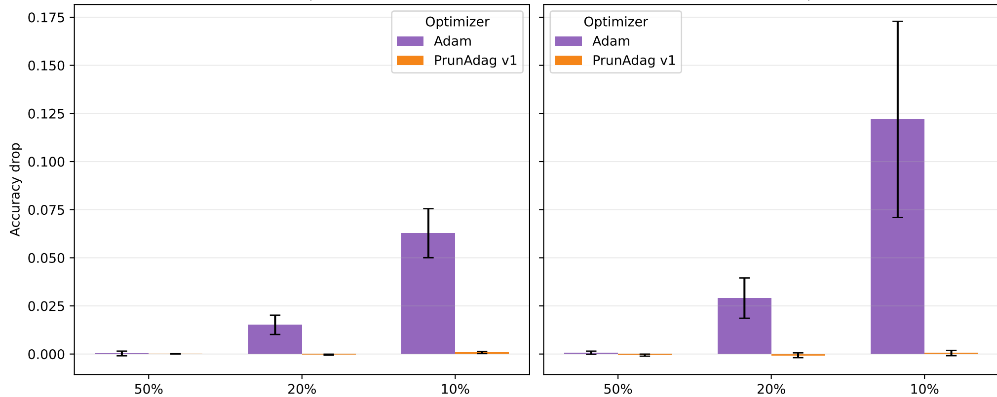
MNIST | MLP
