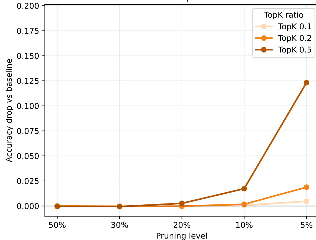
MNIST | MLP
