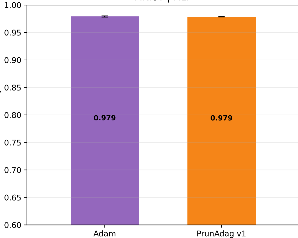
MNIST | MLP
