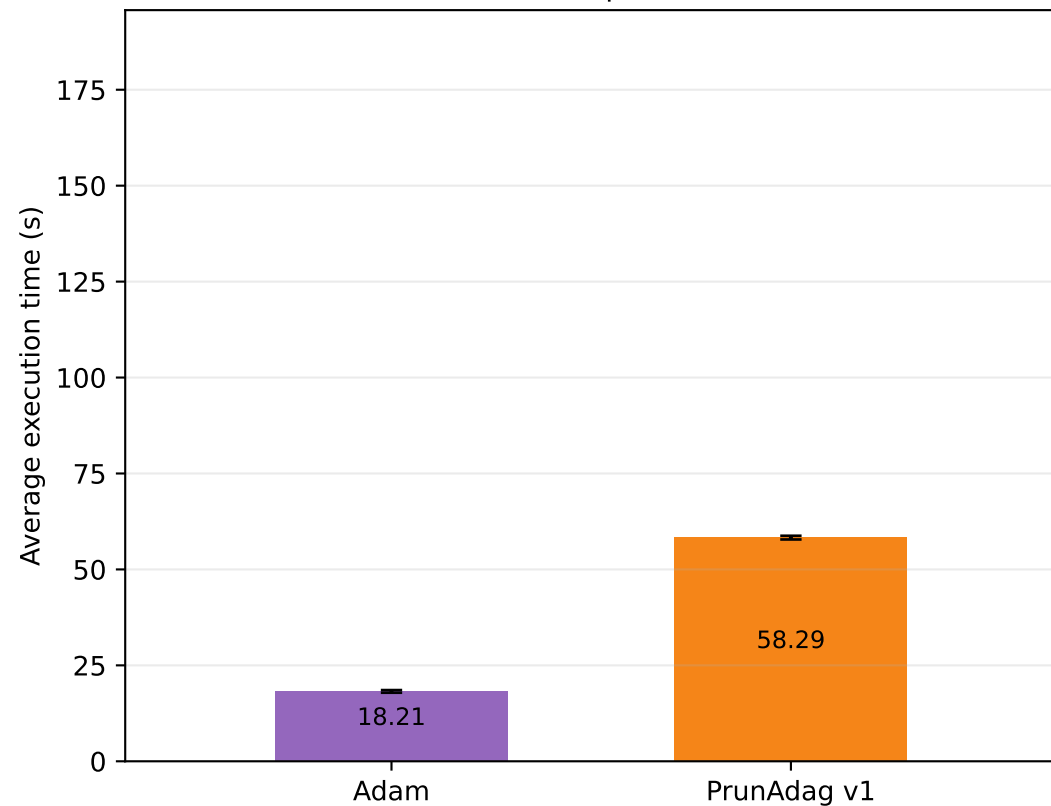
MNIST | MLP
