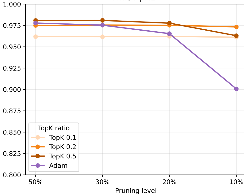
MNIST | MLP
