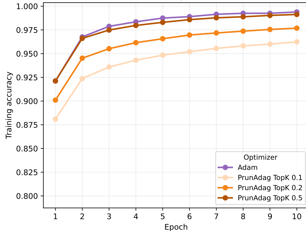
MNIST | MLP
