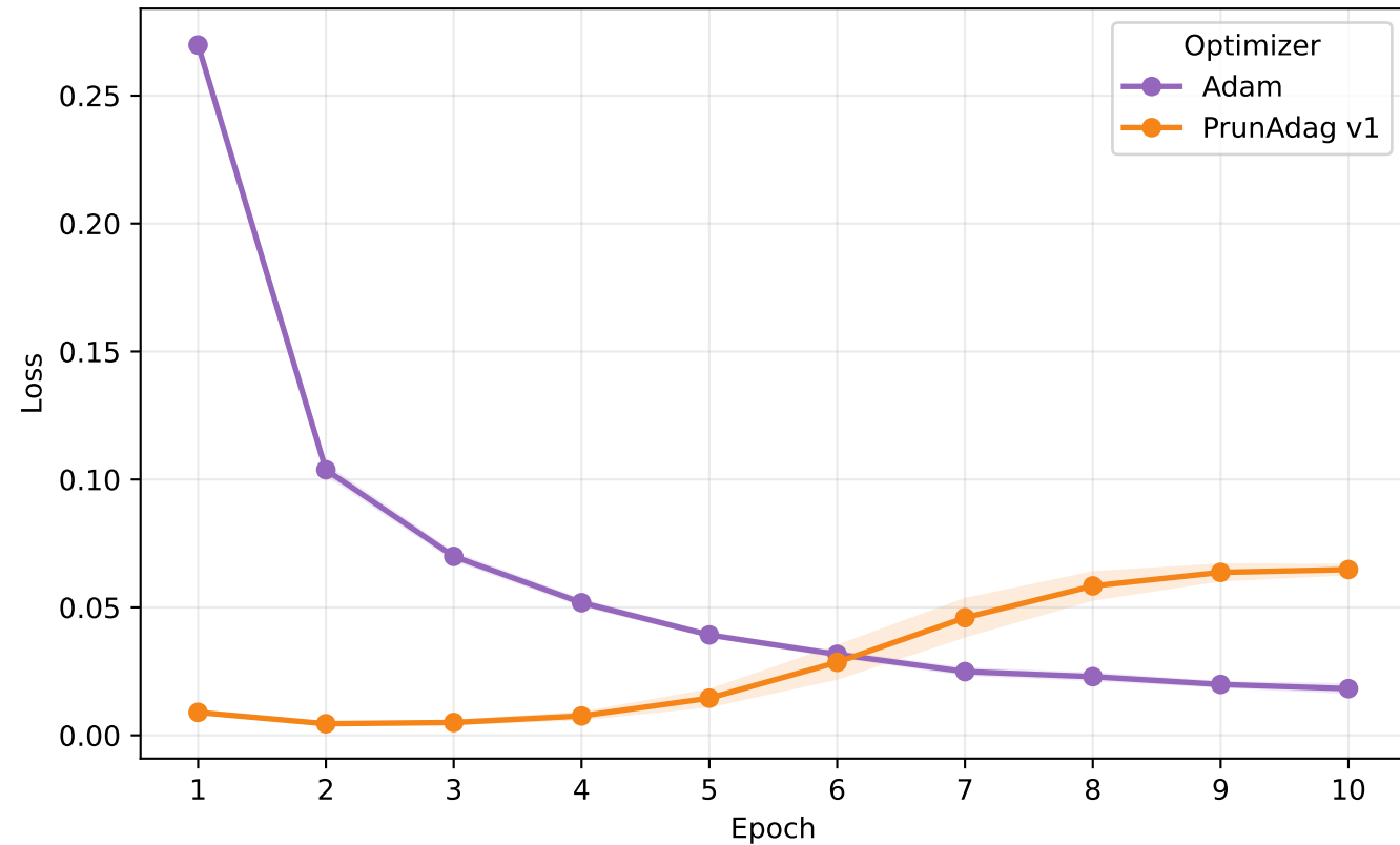
MNIST | MLP
