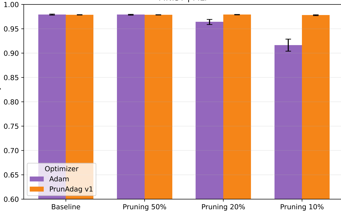
MNIST | MLP
