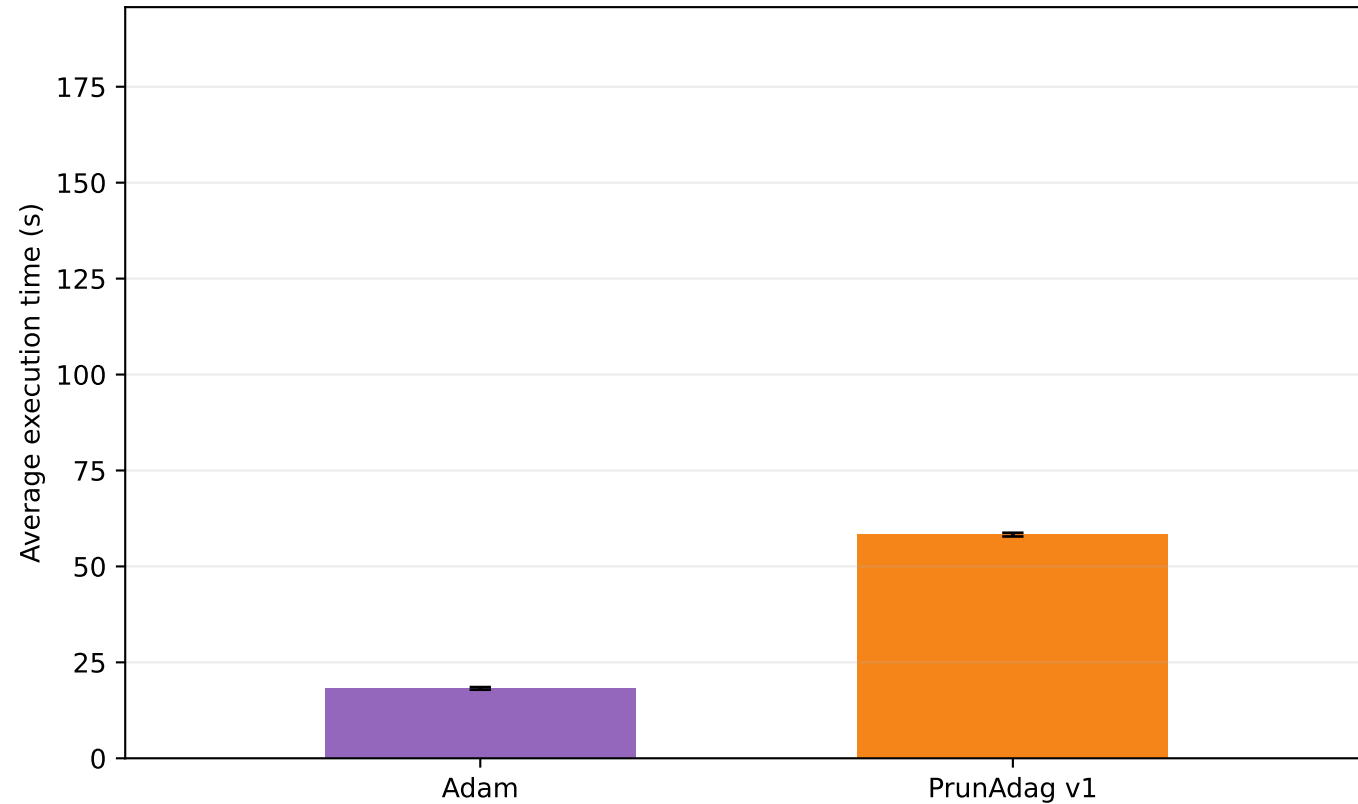
MNIST | MLP
