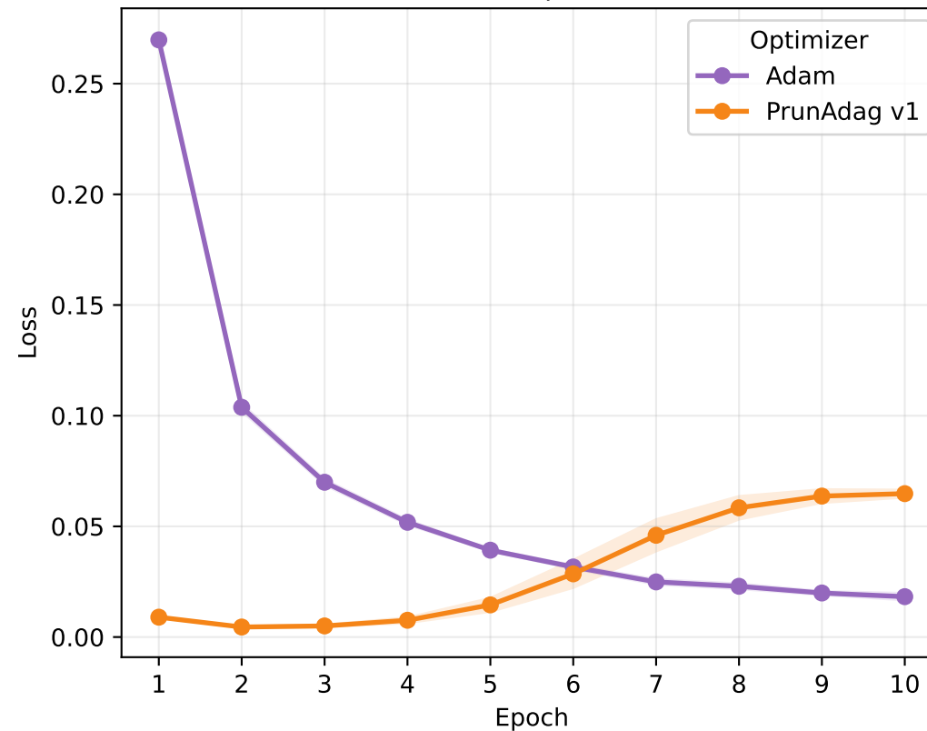
MNIST | MLP
