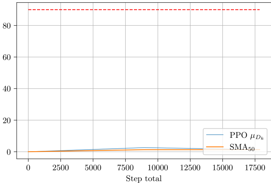
Episodic Reward
