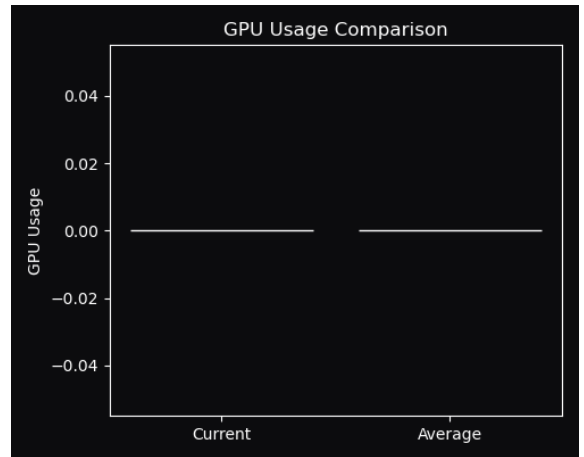
Gpu
