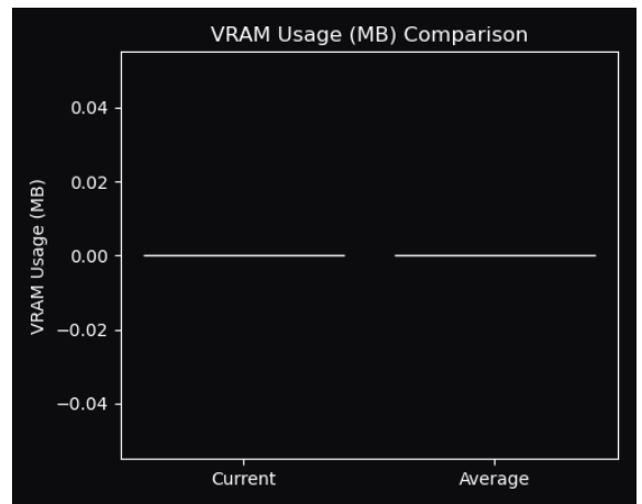
Vram
