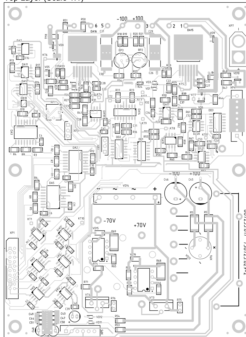
Top Layer (Scale 1:1)
