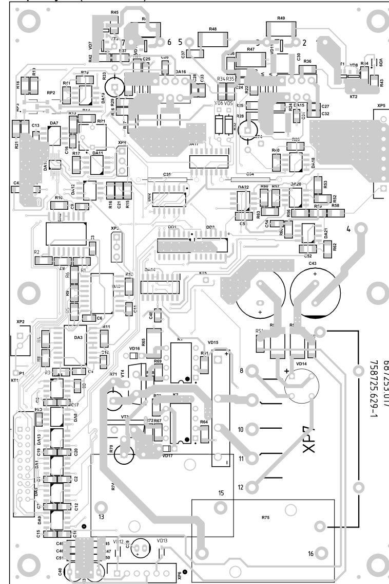
Top Layer (Scale 1:1)
