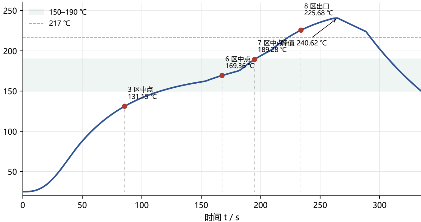
焊接区域中心温度 / °C
