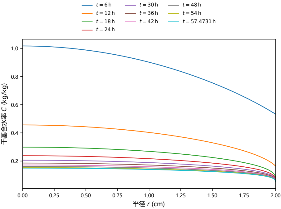
图 6 每 6 h 及结束时刻的径向水分浓度分布
