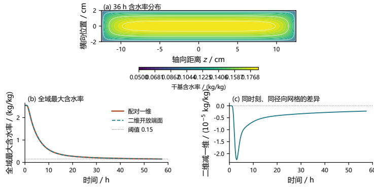
图9 问题三轴对称端面校核。上图为36 h含水率纵剖面，下图为同径向网格的一维与二维最大含水率及差值。
