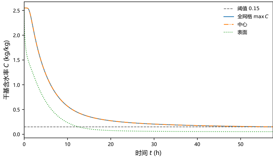
图 5 全域最大水分浓度随时间的变化及干燥阈值
