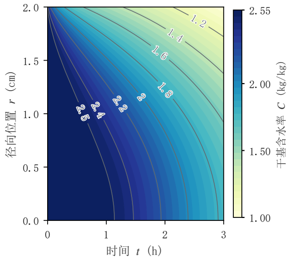
(b) 含水率场
